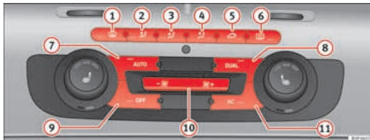
Afb. 135 In het instrumentenpaneel: bedieningselementen van de 2C-Climatronic.
