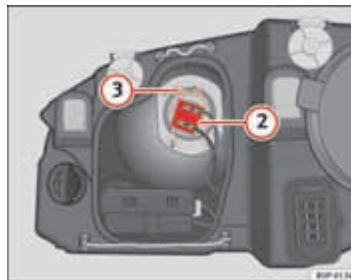
Afb. 190 Dimlicht
