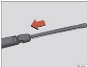
Afb. 173 Wisserblad van de achterraut plaatsen
