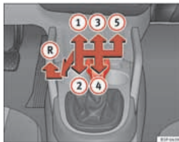
Afb. 143 Deel van de middenconsole: schakelschema van een 5-versnellings schakelbak
