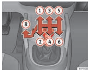
Afb. 144 Deel van de middenconsole: schakelschema van een 6-versnellings schakelbak ▶
