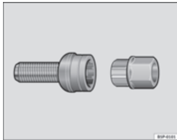
Afb. 184 Wielbout met diefstalbeveiliging
