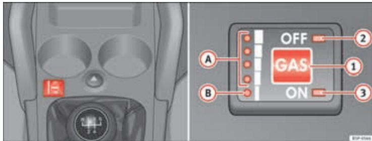
Afb. 140 Middenconsole: schakelaar en controlelampjes van het gassysteem.
