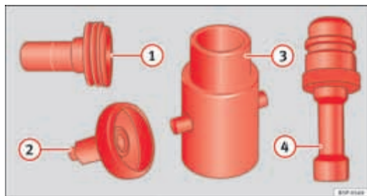
Afb. 162 Overzicht van de adapters voor de LPG-vulmond.
