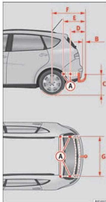
Afb. 158 Bevestigingspunten voor de trekhaak ▶
