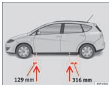
Afb. 180 Steunpunten voor de krik
