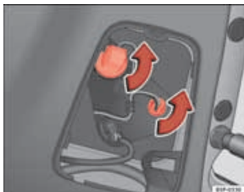
Afbeelding 188 Stadslicht
