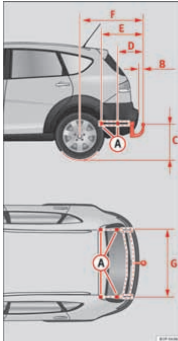
Afbeelding 154 Bevestigingspunten voor de trekhaak
