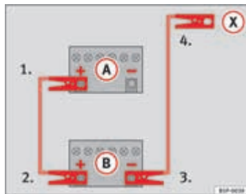
Afbeelding 196 Verbindingschema voor wagens zonder Start-stop-systeem.
