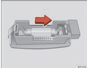
Afbeelding 195 Demontage zonneklepverlichting
