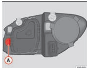
Afbeelding 178 Lampje knipperlicht
