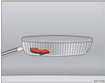
Afbeelding 194 Demontage zonneklepverlichting
