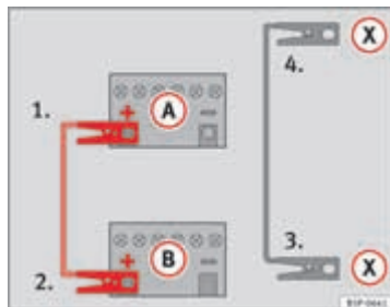
Afbeelding 197 Verbindingschema voor wagens met Start-stop-systeem.
