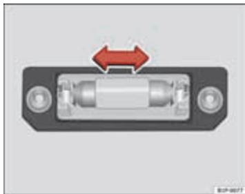
Afbeelding 193 Kentekenplaatverlichting
