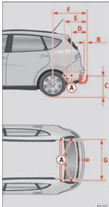
Afbeelding 158 Bevestigingspunten voor de trekhaak
