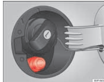
Afbeelding 163 Tankklep open met EURO adapter.
