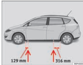
Afbeelding 179 Steunpunten voor de krik
