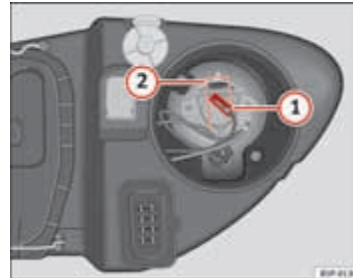
Afbeelding 190 Grootlicht
