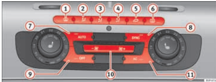
Afbeelding 131 In het dashboard: bedieningselementen van de 2C-Climatronic
