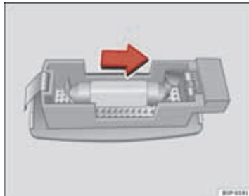
Afbeelding 203 Demontage zonneklepverlichting
