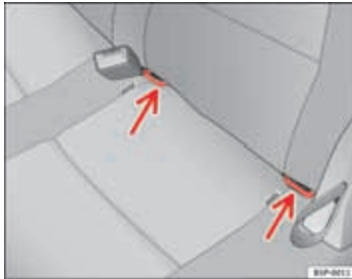
Afbeelding 31 ISOFIX bevestigingsbeugels
