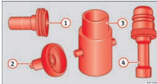
Abbeelding 159 Overzicht van de adapters voor LPG-vulmonden.
