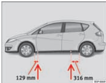
Afbeelding 176 Steunpunten voor de krik
