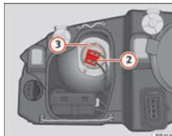
Afbeelding 184 Dimlicht
