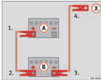
Afbeelding 201 Verbindingschema voor wagens zonder Start-stop-systeem.
