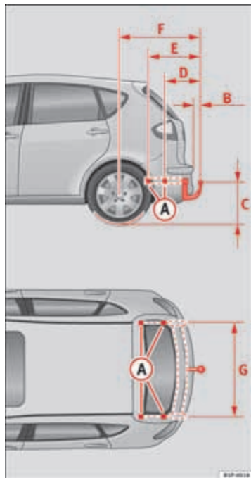
Abbeelding 155 Bevestigingspunten voor de trekhaak
