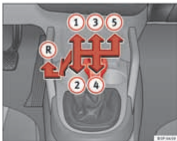
Afbeelding 139 Deel van de middenconsole: schakelschema van een 5-versnellings versnellingsbak
