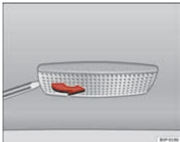
Afbeelding 199 Demon- tage zonneklepverlichting
