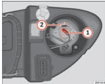
Afbeelding 186 Grootlicht
