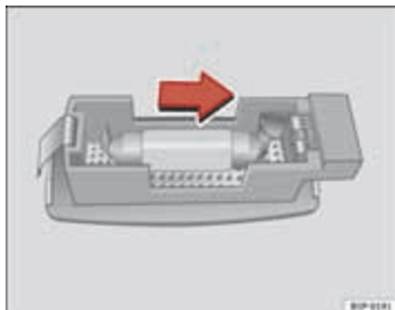
Afbeelding 200 Demon- tage zonneklepverlichting
