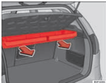
Afbeelding 123 Uitbouwen houder
