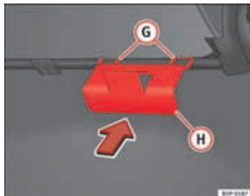
Afbeelding 112 Bevestigingsplaat van het verplaatsbaar opbergvak
