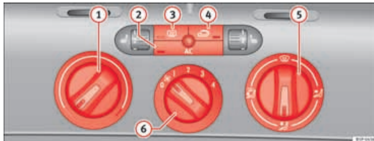
Afbeelding 127 Bedieningselementen van de Climatic in het instrumentenpaneel
