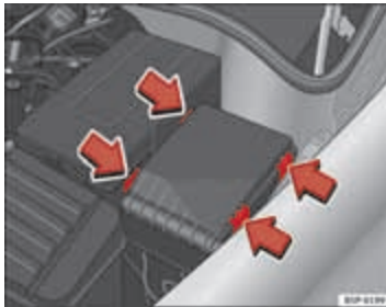
Afbeelding 180 Afdekking van de zekeringenhouder in de motorruimte
