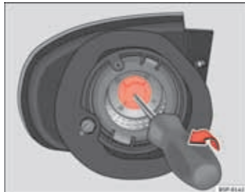
Afbeelding 192 Knipperlicht.
