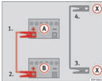
Afbeelding 202 Verbindingschema voor wagens met Start-stop-systeem.
