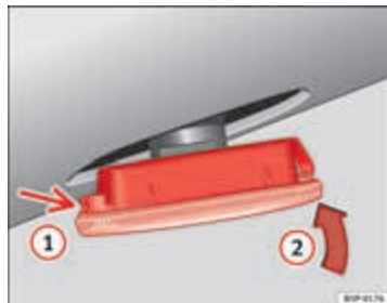
Afbeelding 194 Zijknipperlicht
