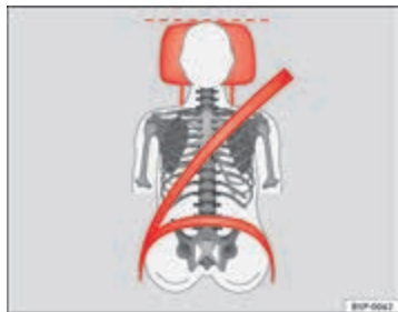
Afbeelding 13 Juist verloop van de gordelband en een juiste stand van de hoofdsteun van voren gezien
