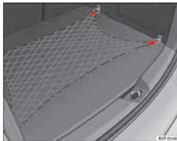
Afbeelding 107 Bagagenet in bagageruimte ▶
