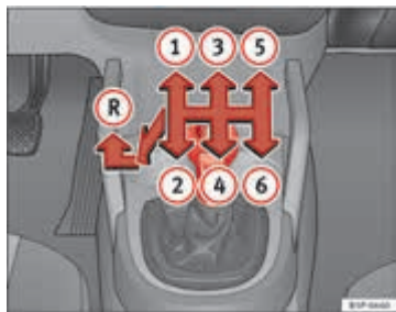
Afbeelding 145 Deel van de middenconsole: schakelschema van een 6-versnellings versnellingsbak
