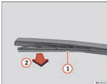
Afbeelding 174 Ruitenwisserblad achterraut vervangen
