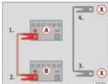
Afbeelding 215 Verbindingschema voor wagens met Start-stop-systeem.
