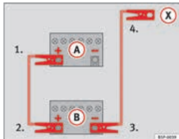
Afbeelding 214 Verbindingschema voor wagens zonder Start-stop-systeem.
