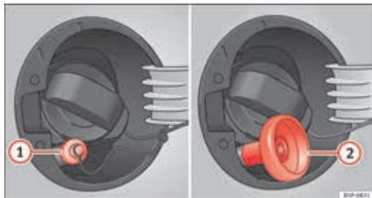
Afbeelding 160 Tankklep open met vulmond van LPG en adapter.
