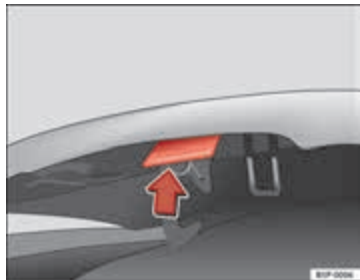
Afbeelding 165 Grendel voor het openen van de motorkap.
