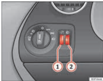
Afbeelding 72 Dashboard: regelaars voor instrumenten- en schakelaarverlichting en lichtbundel-hoogteverstelling
