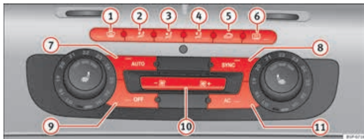
Afbeelding 136 In het dashboard: bedieningselementen van de 2C-Climatronic.
