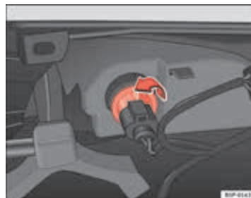
Afbeelding 200 Lichtunit aan de binnenzijde van de bumper
