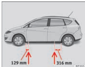
Afbeelding 181 Steunpunten voor de krik
