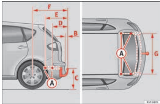
Afbeelding 158 Bevestigingspunten voor de trekhaak
