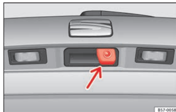
Afb. 217 In de greep van de achterklep: inbouwplaats van achteruitkijkcamera.
