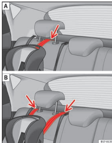
Afb. 33 Bevestigingsband: afstelling en montage volgens de Top Tether-gordel.
