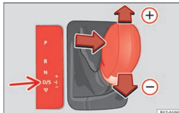
Afb. 169 Middenconsole: schakelen met tiptronic.
