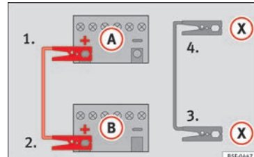
Afb. 78 Verbindingsschema voor wagens met Start-stopstelsysteem.
