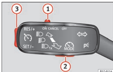
Afb. 175 Links van de stuurkolom: schakelaar en toetsen om de snelheidsbegrenzer te bedienen.
