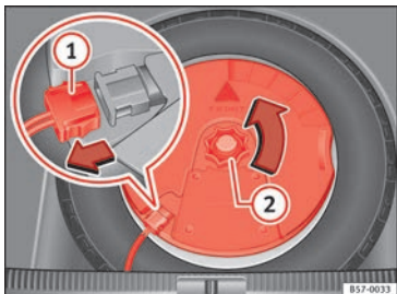
Afb. 231 In de bagageruimte: de subwoofer uitbouwen.
