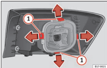
Afb. 111 Bevestigingsclips aan de achterzijde van het achterlicht.
