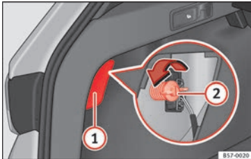
Afb. 110 Bagageruimte: toegang tot de bevestigingsbout van het achterlicht.
