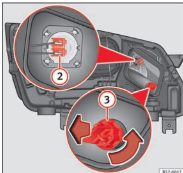
Afb. 107 In de motorruimte: lampje grootlicht ② en lampje knipperlicht ③.
