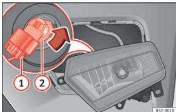
Afb. 109 Mistlamp: fitting uitbouwen
