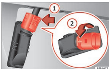
Afb. 115 kentekenverlichting: fitting uitbouwen.
