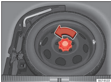
Afb. 230 Noodreservewiel: opgeklapte laadvloer.
