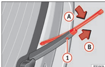
Afb. 81 Ruitenwisserblad van achterruit vervangen.
