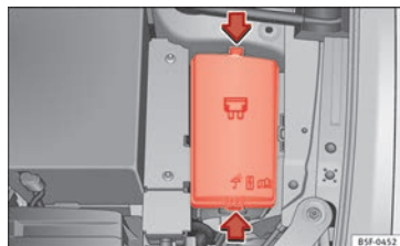
Afb. 103 In de motorruimte: deksel van de zekeringenhouder.
