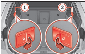
Afb. 146 In de bagageruimte: hendels voor de ontgrendeling op afstand van de linkerzijde ① en rechterzijde ② van de achterste rugleuning.
