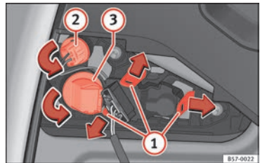
Afb. 113 Fitting uitbouwen.
