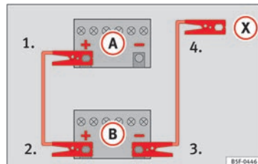
Afb. 77 Verbindingsschema voor wagens zonder Start-stopstelsysteem.
