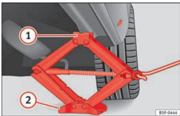
Afb. 74 Langsligger: plaatsing van de wagenkrik.
