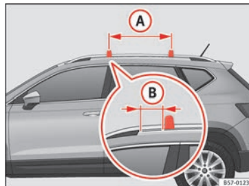
Afb. 162 Bevestigingspunten voor de reling van het dakdragersysteem.
