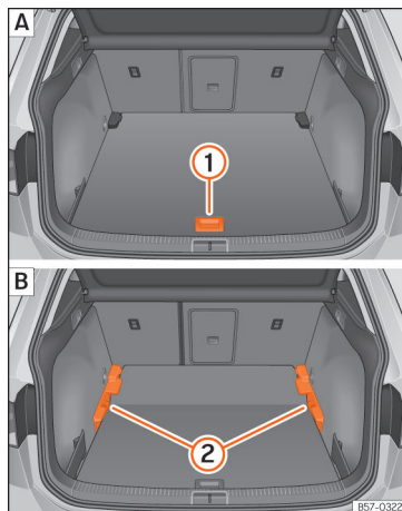
Afb. 180 Verstelbare bodem van de bagageruimte: A hoge stand; B lage stand.
