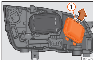
Afb. 110 In de motorruimte: de afdekking verwijderen.
