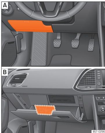
Afb. 67 [A] Stuur links: afdekking van de zekeringenhouder in het dashboard aan bestuurderszijde. [B] Stuur rechts: zekeringenhouder achter het dashboardkastje.
