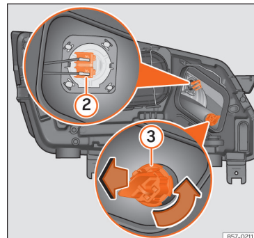
Afb. 111 In de motorruimte: lampje grootlicht ② en lampje knipperlicht ③.
