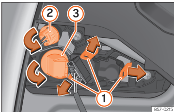
Afb. 117 Fitting uitbouwen.
