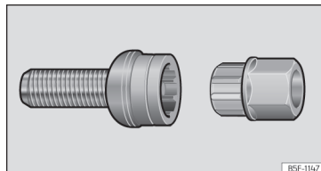
Afb. 76 Wielbout met diefstalbeveiliging, voorzien van dop en adapter.
