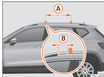
Afb. 182 Bevestigingspunten voor de reling van het dakdragersysteem.
