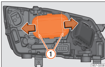
Afb. 108 In de motorruimte: de afdekking verwijderen.
