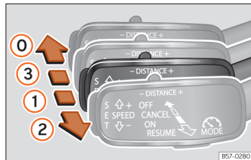
Afb. 261 Links van de stuurkolom: derde hendel om de automatische afstandsregeling te bedienen.
