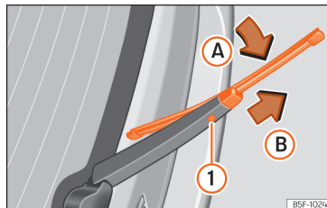
Afb. 86 Ruitenwisserblad van achterruit vervangen.
