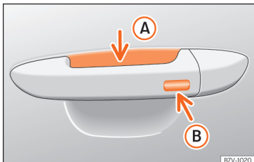
Afb. 140 Sluit- en startsysteem zonder sleutel Keyless Access: sensoroppervlak (A) voor het ontgrendelen aan de binnenzijde van de portiergreep van het portier en sensoroppervlak (B) voor het vergrendelen aan de buitenzijde van de portiergreep.
