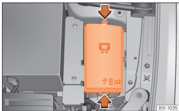
Afb. 107 In de motorruimte: deksel van de zekeringenhouder.
