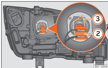
Afb. 109 In de motorruimte: lampje dimlicht.
