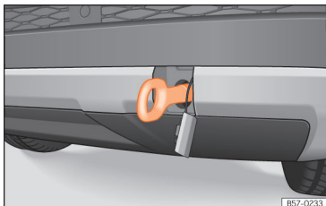
Afb. 104 Aan de rechterzijde van de achterbumper: vastgeschroefd sleepoog.
