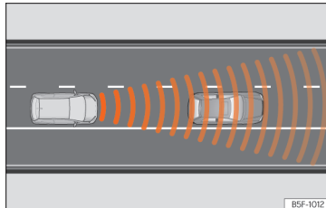
Afb. 258 Detectiegebied.
