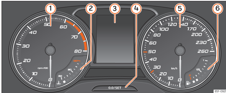
Afb. 123 Instrumentenpaneel, in het dashboard.
