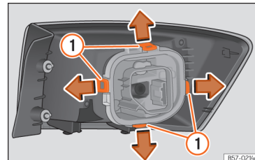
Afb. 115 Bevestigingslippen aan de achterzijde van het achterlicht.
