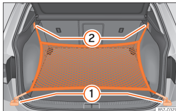
Afb. 140 In de bagageruimte: ringen ① en haken ② voor het vasthaken van de nettas.
