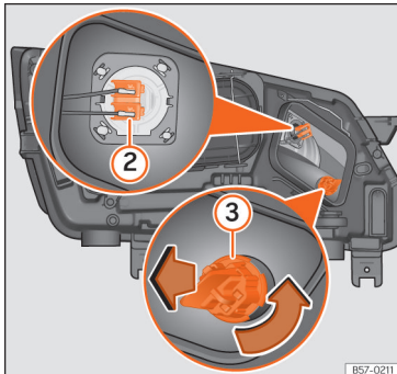
Afb. 58 In de motorruimte: lampje grootlicht ② en lampje knipperlicht ③.
