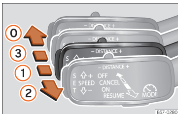
Afb. 264 Links van de stuurkolom: derde hendel voor bediening van ACC.
