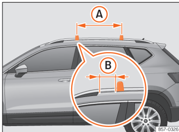
Afb. 144 Bevestigingspunten voor de reling van het dakdragersysteem.
