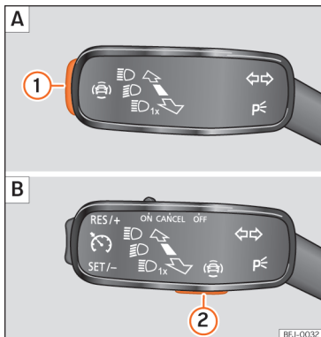
Afb. 81 In de knipperlicht- en grootlichthendel: toets voor de bestuurdershulpsystemen (naargelang het model).
