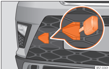
Afb. 47 Aan de rechterzijde van de voorbumper: de afdekking verwijderen.
