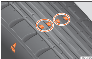
Afb. 318 Bandenprofiel: slijtagemerkttekens.
