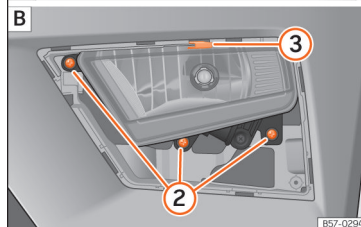
Afb. 59 Mistlamp: rooster verwijderen. »
