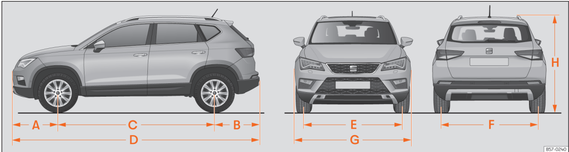
Afb. 323 Afmetingen
