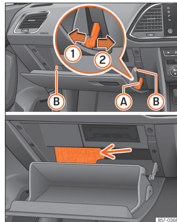
Afb. 52 Dashboardkastje (stuur rechts): toegang tot de zekeringenhouder.
