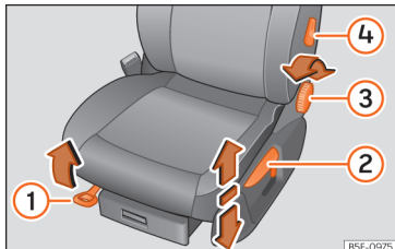
Afb. 124 Voorstoelen: handmatige instelling van de stoel.
