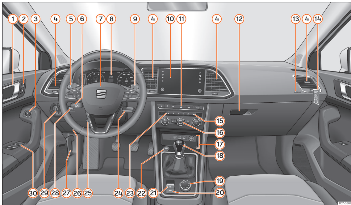
Afb. 68 Bestuurdersruimte.
