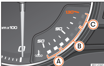
Afb. 77 Analoog instrumentenpaneel: koelvloeistoftemperatuurmeter.
