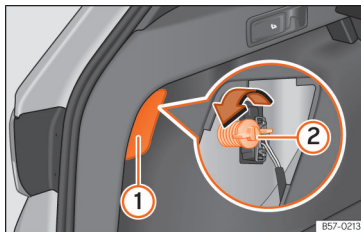
Afb. 61 Bagageruimte: toegang tot de bevestigingsbout van het achterlicht.
