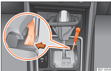
Afb. 246 Keuzehendel: noodontgrendeling in de parkeerstand.
