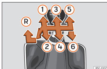
Afb. 242 Schema van een handmatige versnelling met 5 of 6 standen.
