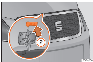
Afb. 309 Hendel onder de motorkap.
