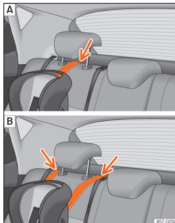
Afb. 30 Zitplaatsen achterin: afstelling en montage volgens de Top Tether-gordel.
