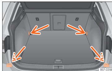
Afb. 138 In de bagageruimte: bevestigingsogen.
