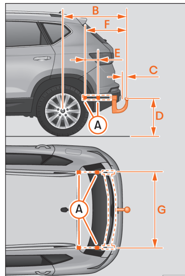
Afb. 302 Maten en bevestigingspunten voor het achteraf inbouwen van een trekhaak.
