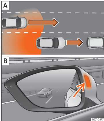
Afb. 180 Schematische weergave: A Situatie van het inhalen met verkeer aan de achterzijde. B Indicatie van de rijstroomwisselassistent in de buitenspiegel links.
