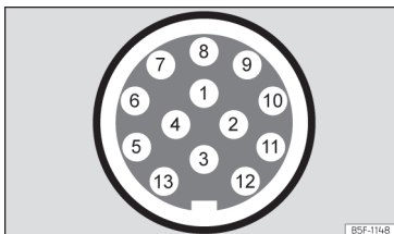
Afb. 202 Schematische weergave: toewijzing van de pinnen van het stopcontact voor de aanhangwagen.
