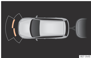
Afb. 194 Weergave van de parkeerhulp op het scherm met aangekoppelde aanhangwagen.
