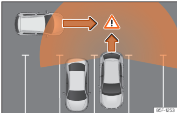
Afb. 182 Schematische weergave van de uitparkeerhulp: bewaakte zone rond de wagen die aan het uitparkeren is.
