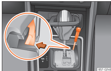
Afb. 156 Keuzehendel: noodontgrendeling in de parkeerstand.
