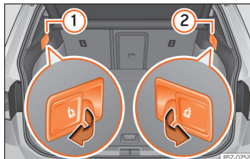
Afb. 114 In de bagageruimte: hendels voor de ontgrendeling op afstand van de linkerzijde 1 en rechterzijde 2 van de achterste rugleuning.
