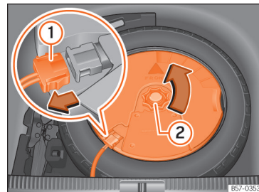
Afb. 224 In de bagageruimte: subwoofer uitbouwen.
