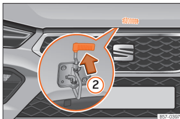
Afb. 209 Hendel onder de motorkap.
