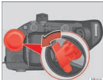
Afb. 221 Lampje knipperlicht
