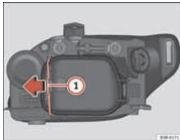
Afb. 222 Lampje van het stadslicht
