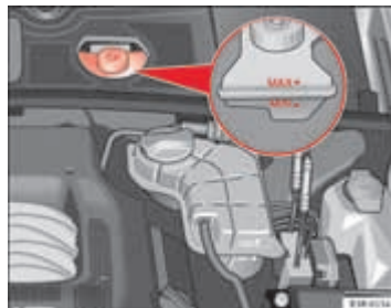
Afb. 187 Motorruimte: markeringen op het remvloeistofreservoir
