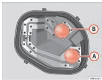
Afb. 228 Positie van de gloeilampjes op de fittingplaat: Voorbeeld: buitenste linkerachterlicht
