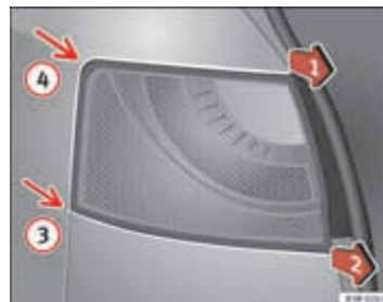
Afb. 226 Uitbouwen van achterlicht in zijpaneel ►
