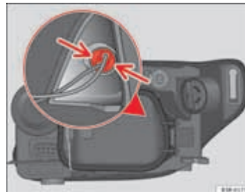
Afb. 213 Stadslicht (buitenzijde wagen)
