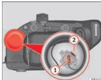
Afb. 209 Grootlicht
