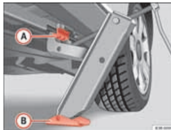
Afb. 197 Wiel verwisselen: Krik
