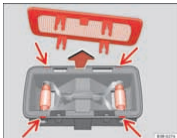
Afb. 238 Licht bagageruimte
