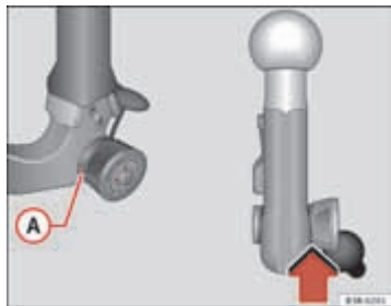
Afb. 168 Afneembare trekhaak: Veiligheidscontrole
