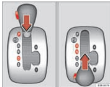
Afb. 156 Keuzehendelvergrendeling
