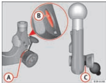
Afb. 165 Afneembare trekhaak: Stang met kogelkop
