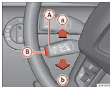
Afb. 152 Bedieningselementen van het snelheidsregelsysteem
