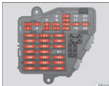
Afb. 203 Algemene afbeelding van de zekeringssteun aan de linkerkant van het dashboard: Zekeringen (zonder deksel)
