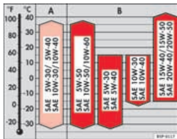
Afb. 178 Oliesoorten volgens temperatuur
