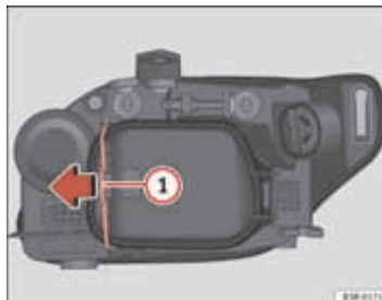
Afb. 214 Stadslicht (binnenzijde wagen)
