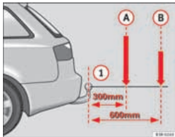
Afb. 161 Principeafbeelding van de gewichtsverdeling van aanbouwdelen en accessoires
