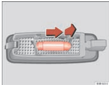
Afb. 242 Demontage zonneklepverlichting
