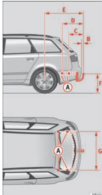
Afb. 172 Bevestigingspunten voor de trekhaak ▶
