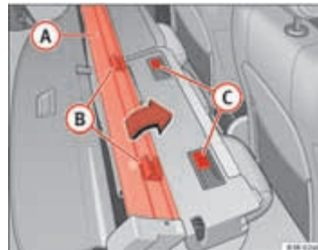
Afb. 123 Bagageruimte-afdekking/scheidingsnet inbouwen
