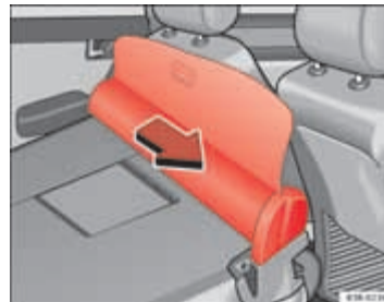
Afb. 122 Bagageruimte-afdekking/scheidingsnet uitbouwen
