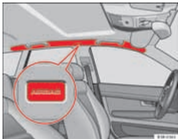
Afb. 25 Inbouwplaats van de hoofdairbags aan de linkerwagzijde
