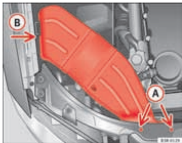
Afb. 204 Luchtgeleidingskap aan de rechterkant van de wagen
