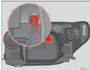
Afb. 223 Lampje van het stadslicht
