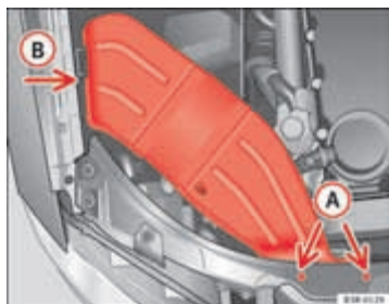
Afb. 217 Luchtgeleidingskap aan de rechterkant van de wagen
