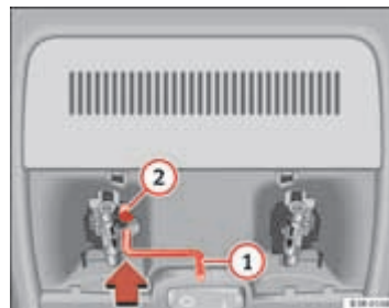
Afb. 84 Deel van de hemelbekleding: Slinger voor noodbediening
