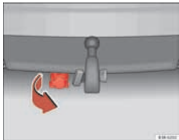
Afb. 169 Achterbumper: Aanhangwagenstopcontact naar beneden zwenken
