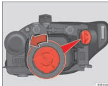
Afb. 207 Lampje knipperlicht
