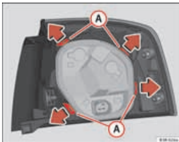
Afb. 227 Bevestigingslippen achter op achterlicht
