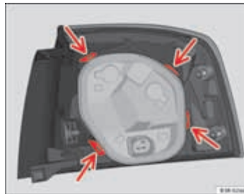
Afb. 229 Fittingplaat in achterlicht bevestigen
