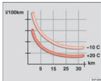
Afb. 110 Brandstofverbruik in l/100 km bij twee verschillende omgevings-temperaturen
