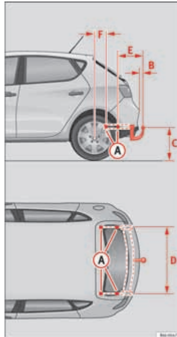
Afb. 111 Bevestigingspunten voor de trekhaak ▶
