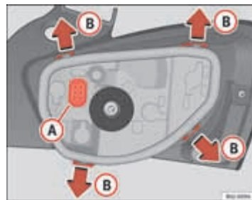
Afb. 145 Vervanging lampjes achterlichten
