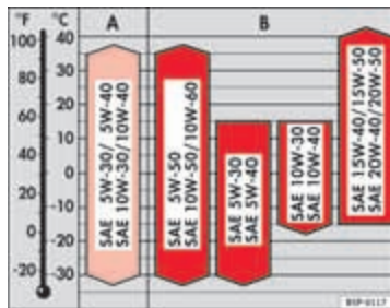
Afb. 115 Oliesoorten volgens temperatuur
