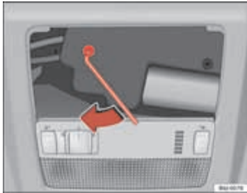
Afb. 51 Noodaansturing panoramisch dak/kanteldak
