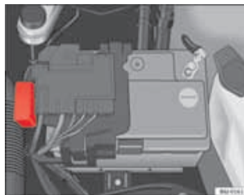
Afb. 132 Zekeringen in de motorruimte
