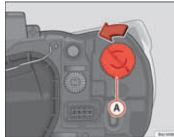
Afbeelding 152 Knipperlicht enkele koplamp
