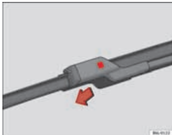
Afbeelding 138 Ruitenwischerbladen voorruit vervangen
