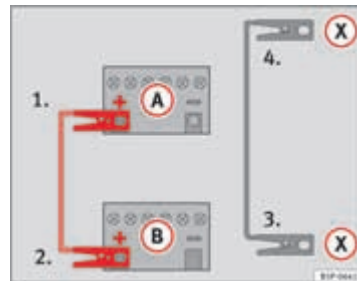
Afbeelding 179 Verbindingschema voor wagens met Start-stop-systeem.
