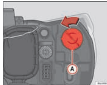
Afbeelding 163 Knipperlicht ▶
