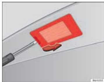
Afbeelding 174 Kentekenverlichting uitbouwen.
