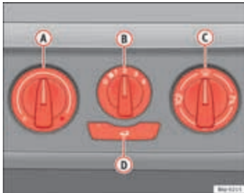
Afbeelding 100 Op het dashboard: bedienings-elementen van de verwarming
