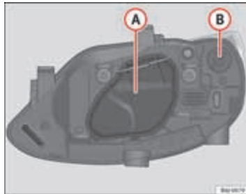
Afbeelding 151 Enkele koplamp
