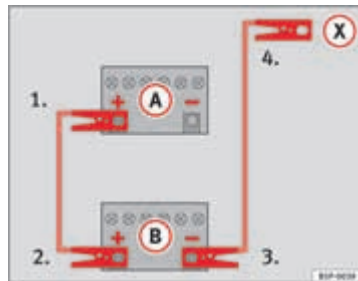
Afbeelding 178 Verbindingschema voor wagens zonder Start-stop-systeem.
