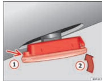
Afbeelding 173 Zijknipperlichten
