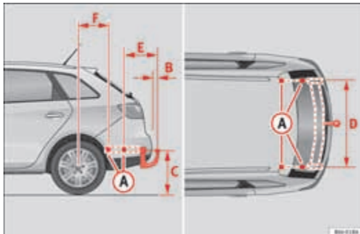
Afbeelding 126 Bevestigingspunten voor de trekhaak
