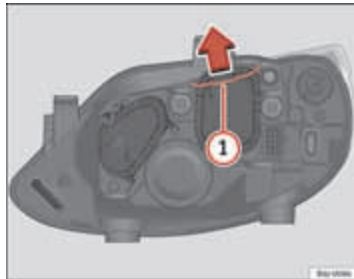
Afbeelding 161 Dimlicht
