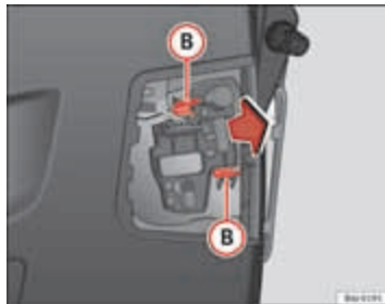
Afbeelding 172 Demontage fitting
