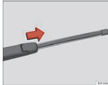
Afbeelding 139 Wisserblad van de achterruit verwijderen
