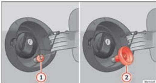
Afbeelding 128 Tankklep open met vulmond van LPG en adapter.
