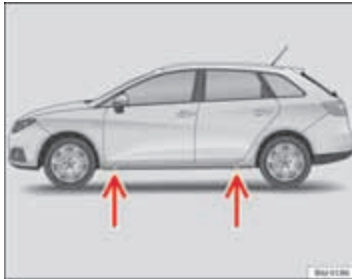
Afbeelding 146 Steunpunten voor de krik
