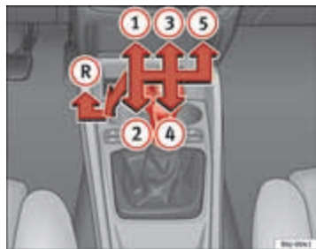
Afbeelding 111 Middenconsole: schakelschema van een 5-versnellings handgeschakelde versnellingsbak
