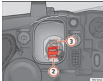
Afbeelding 162 Dimlicht
