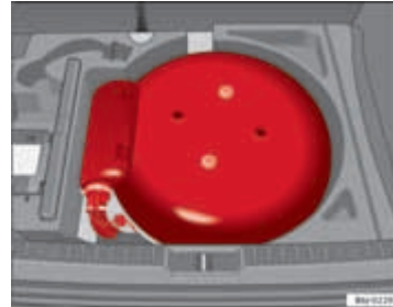
Afbeelding 121 LPG-tank in uitsparing voor reservewiel.
