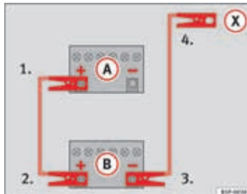
Afbeelding 168 Verbindingsschema voor wagens zonder Start-stop-systeem.
