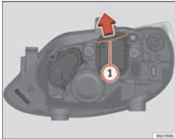
Afbeelding 153 Dimlicht
