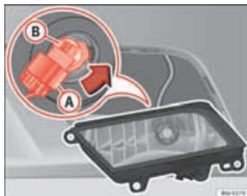
Afbeelding 160 Mis- tlamp
