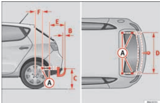
Afbeelding 118 Bevestigingspunten voor de trekhaak
