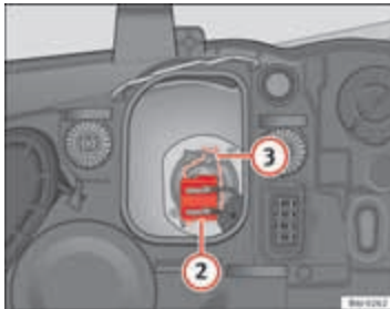
Afbeelding 154 Dimlicht
