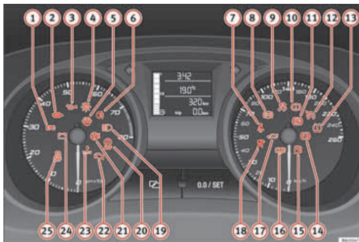
Afbeelding 38 Instrumentenpaneel met waarschuwing- en controlelampjes. Enkele van de hier genoemde waarschuwing- en controlelampjes horen bij bepaalde type-uitvoeringen of zijn onderdeel van meeruitvoeringen
