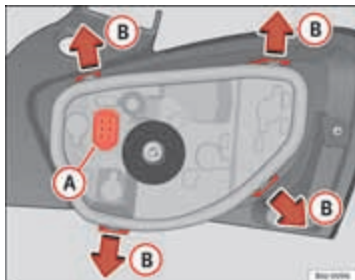
Afbeelding 162 Vervanging lampjes achterlichten
