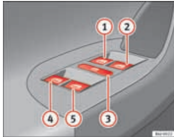
Afbeelding 51 Deel van het bestuurdersportier: bedieningselementen van voorste en achterste ruiten
