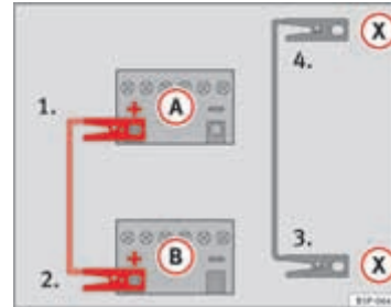
Afbeelding 169 Verbindingsschema voor wagens met Start-stop-systeem.
