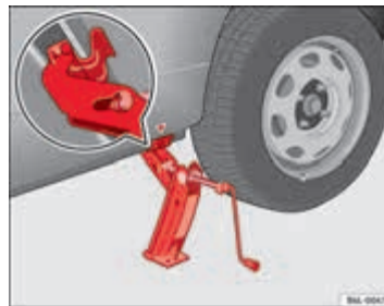
Afbeelding 150 Plaatsen van de krik
