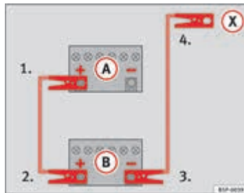
Afbeelding 188 Verbindingschema voor wagens zonder start-stop-systeem.
