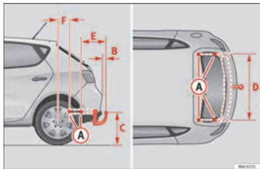
Afbeelding 129 IBIZA / IBIZA SC: Bevestigingspunten voor de trekhaak
