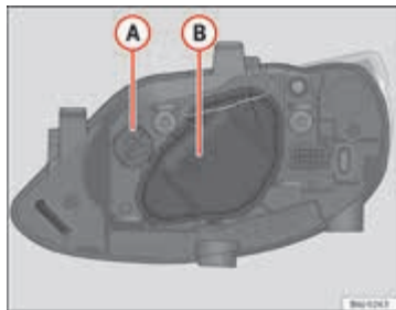
Afbeelding 168 Lampjes van AFS koplamp
