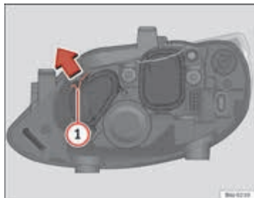
Afbeelding 163 Grootlicht
