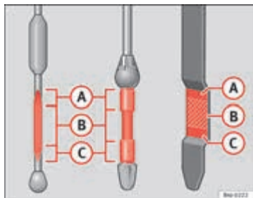
Afbeelding 136 Oliepeil-stok
