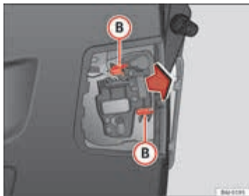
Afbeelding 182 Demontage fitting
