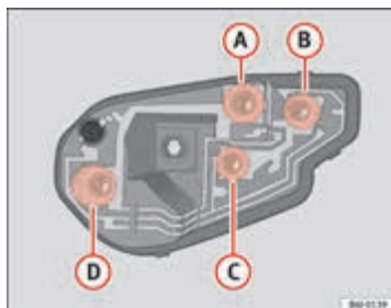
Afbeelding 175 Rechterlampje
