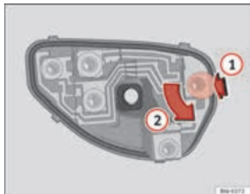
Afbeelding 178 Vervanging lampjes achterlichten
