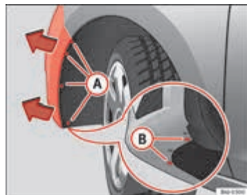
Afbeelding 172 Mis- tlamp: toegang tot de connector en de fitting
