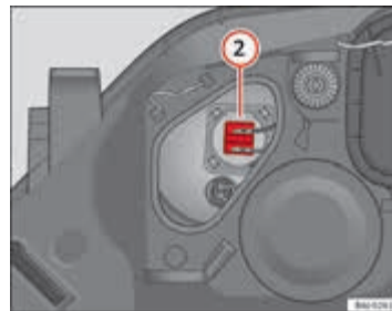
Afbeelding 164 Grootlicht
