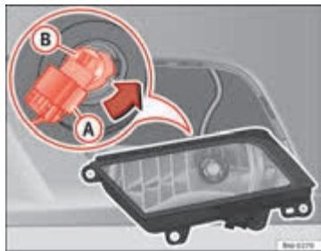
Afbeelding 173 Mistlamp
