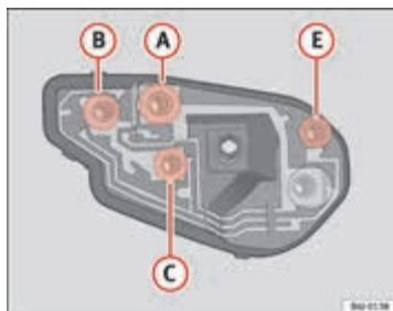
Afbeelding 174 Linkerlampje
