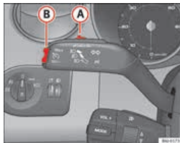
Afbeelding 125 Knipperlicht- en grootlichthendel: schakelaar en tuimelschakelaar voor het snelheidsregelsysteem
