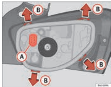
Afbeelding 177 Vervanging lampjes achterlichten
