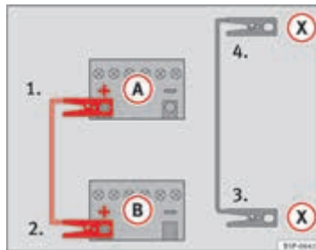
Afbeelding 189 Verbindingschema voor wagens met start-stop-systeem.
