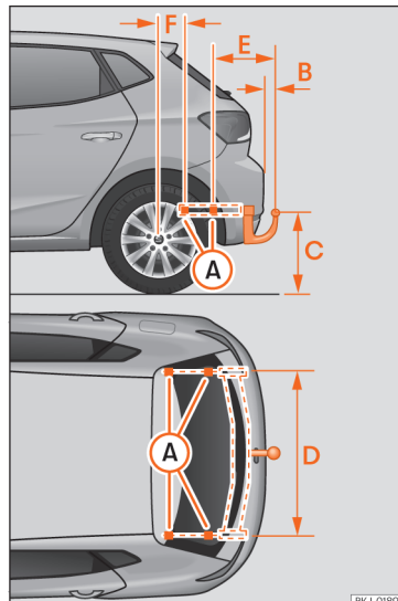
Afb. 264 Bevestigingspunten voor de trekhaak.
