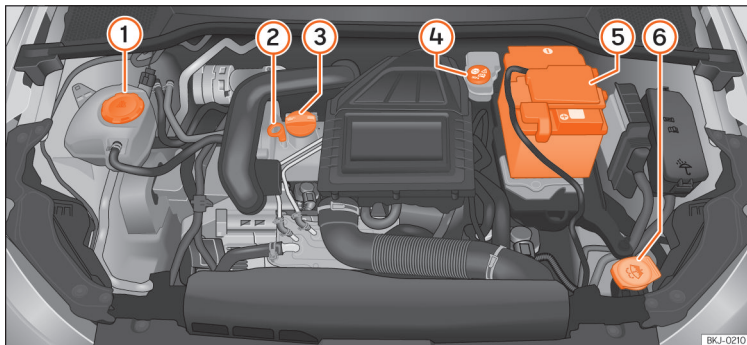
Afb. 269 Afbeelding met de plaats van de elementen.
