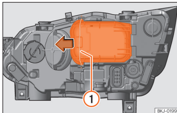
Afb. 104 In de motorruimte: de afdekking verwijderen.
