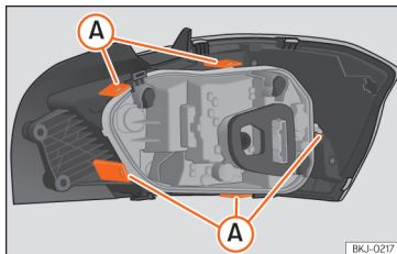
Afb. 109 Bevestigingslippen aan de achterzijde van het achterlicht.
