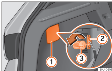
Afb. 108 Bagageruimte: toegang tot de bevestigingsbout van het achterlicht.
