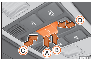
Afb. 141 In de hemelbekleding: toets van het glazen dak.
