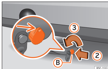
Afb. 260 Slot deblokkeren
