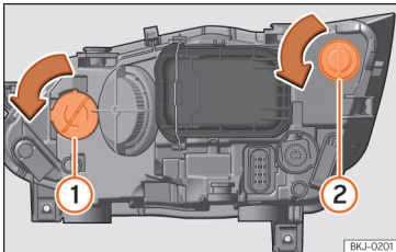
Afb. 106 In de motorruimte: lampje knipperlicht ① en lampje DRL-licht (daglicht) ②.
