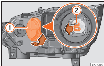
Afb. 103 In de motorruimte: lampje grootlicht.
