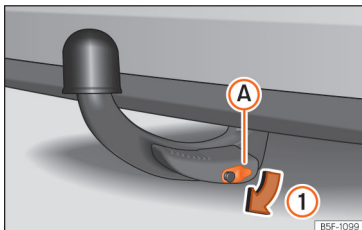
Afb. 259 Het deksel van het slot verwijderen
