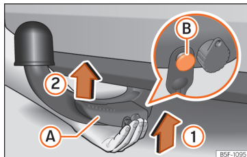
Afb. 255 Afneembare kogelkop plaatsen / ontgrendelbout in uitgeschoven toestand
