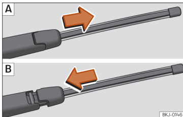
Afb. 84 Wisserblad van de achterraut verwijderen en plaatsen.
