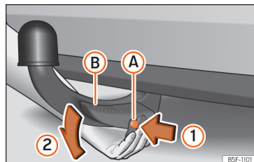
Afb. 261 De afneembare kogelkop losmaken
