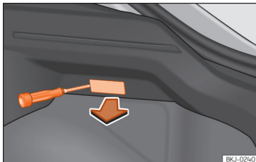
Afb. 112 Bagageruimteverlichting.
