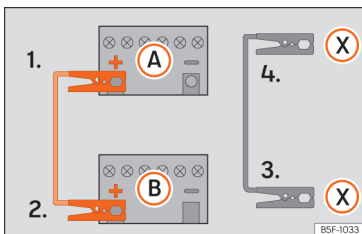
Afb. 81 Verbindingsschema voor wagens met start-stopsysteem.
