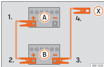
Afb. 80 Verbindingsschema voor wagens zonder start-stopsysteem.
