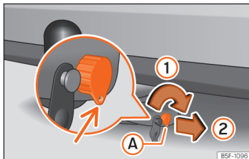
Afb. 256 Slot blokkeren
