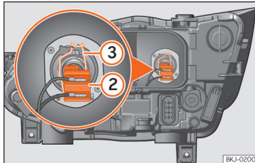
Afb. 105 In de motorruimte: lampje dimlicht.
