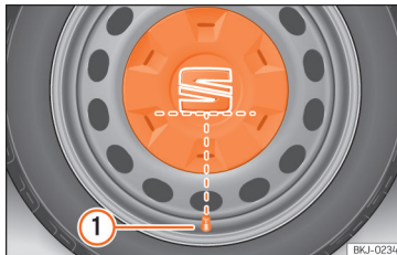
Afb. 71 Juiste plaatsing van de centrale wioldop voor stalen velgen.
