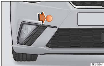
Afb. 99 Voorbumper rechts: de afdekking verwijderen.
