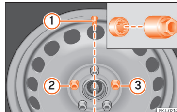
Afb. 75 Wiel verwisselen: ventiel van de band ① en montageplaats van de antidiefstalbout ② of ③.
