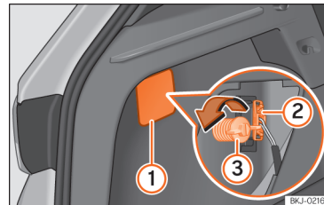
Afb. 60 Bagageruimte: toegang tot de bevestigingsbout van het achterlicht.
