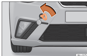
Afb. 48 Rechterzijde van de voorbumper: vastgeschroefd sleepoog.
