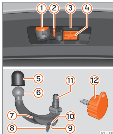
Afb. 251 Steun van de trekhaak voor aanhangwagen / trekhaak / sleutel
