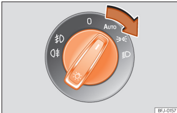
Afb. 105 Dashboard: lichtschakelaar.
