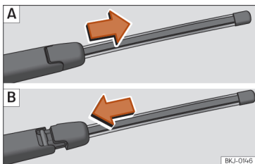
Afb. 44 Wisserblad van de achterruit verwijderen en plaatsen.
