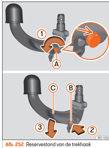
Afb. 252 Reservestand van de trekhaak
