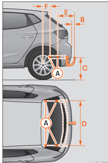
Afb. 260 Maten en bevestigingspunten voor het achteraf inbouwen van een trekhaak.
