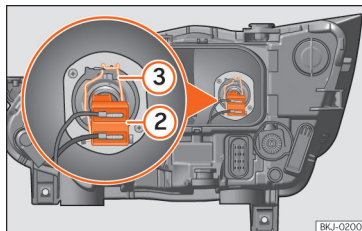
Afb. 56 In de motorruimte: lampje van het dimlicht.
