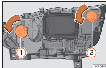
Afb. 57 In de motorruimte: lampje knipperlicht ① en lampje DRL-licht (daglicht) ②.
