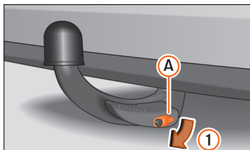
Afb. 258 De trekhaak demonteren
