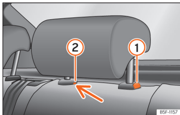
Afb. 122 Hoofdsteun achterin: verwijderen.
