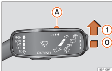
Afb. 114 Ruitenwisserhendel: regensensor A afstellen.
