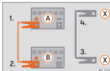
Afb. 46 Verbindingsschema voor wagens met Start-stopsysteem.
