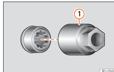
Afb. 37 Wielbout met diefstalbeveiliging, voorzien van dop en adapter.
