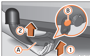
Afb. 254 Plaatsing van de trekhaak. Stap 1
