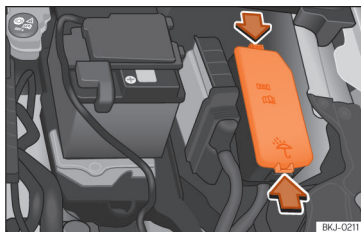
Afb. 52 In de motorruimte: afdekking van de zekeringenhouder.
