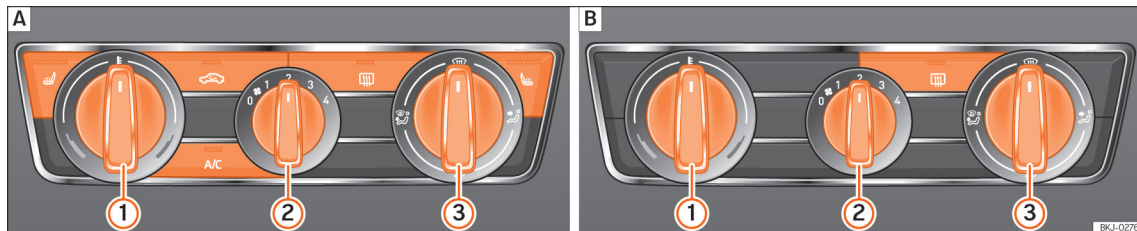
Afb. 139 In de middenconsole: A bedieningselementen van de handbediende airconditioning; B bedieningselementen van het verwarmings- en ventilatiesysteem.
