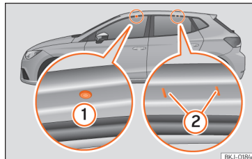
Afb. 131 Bevestigingspunten voor de reling van het dakdragersysteem.
