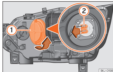
Afb. 54 In de motorruimte: lampje van het grootlicht.
