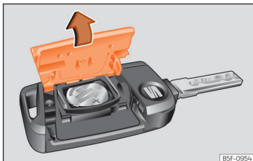
Afb. 87 Wagensleutel: openen van het deksel van batterijvak.
