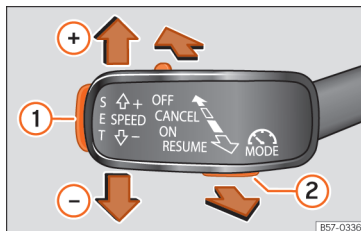
Afb. 227 Links van de stuurkolom: toetsen voor bediening van de snelheidsbegrenzer.
