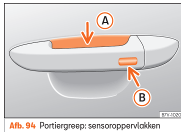
Afb. 94 Portiergreep: sensoroppervlakken
