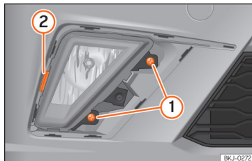
Afb. 59 Mistlamp: fitting uitbouwen
