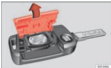
Afbeelding 46 Wagen- sleutel: openen van het deksel van batterijcom- partiment.
