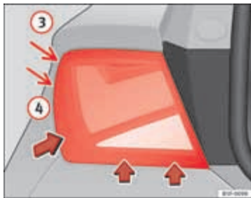
Afbeelding 144 Uitbouwen van achterlicht in zijpaneel
