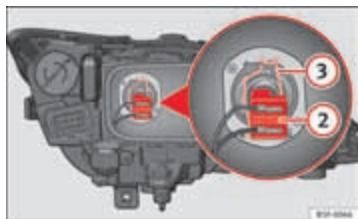
Afbeelding 134 Dimlicht
