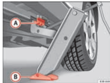
Afbeelding 124 Langsligger: plaatsing van de wagenkrik
