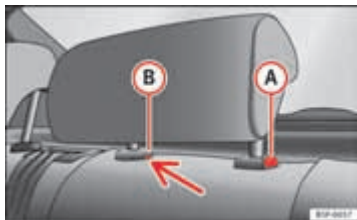
Afbeelding 74 Hoofdsteun midden achter: de-blokkering
