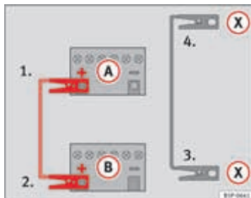
Afbeelding 127 Aansluit-schema voor wagens met start/stop-systeem.
