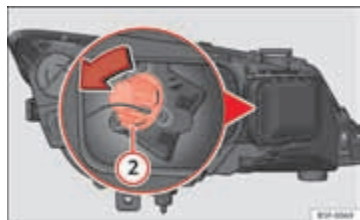
Afbeelding 137 Lampje knipperlicht
