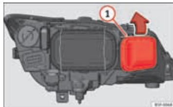
Afbeelding 138 Lampje van het grootlicht
