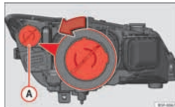
Afbeelding 135 Lamp daglicht
