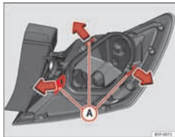
Afbeelding 145 Bevestigingsstrips achter op achterlicht
