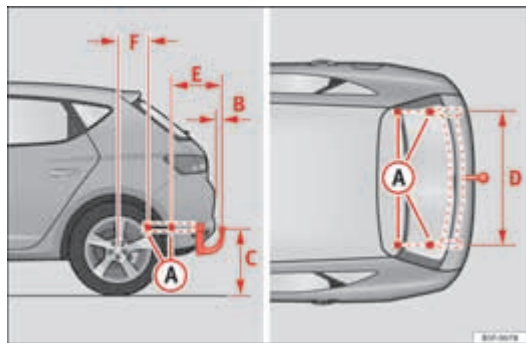
Afbeelding 105 Bevestigingspunten voor de trekhaak
