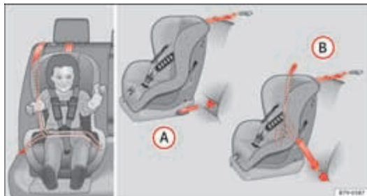
Afbeelding 31 Op de achterbank: de afbeelding (A) toont de basisbevestiging van het bevestigingssysteem voor kinderen met de bevestigingsringen onderaan en de bevestigingsgordel bovenaan. Afbeelding (B) toont de bevestiging van het bevestigingssysteem voor kinderen met de veiligheidsgordel van de wagen.
