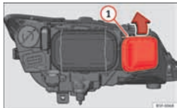
Afbeelding 136 Lampje knipperlicht
