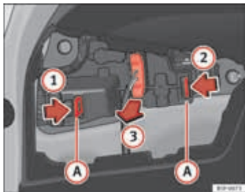
Afbeelding 147 Fitting uitbouwen
