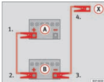
Afbeelding 126 Aansluit-schema voor wagens zonder start/stop-systeem.
