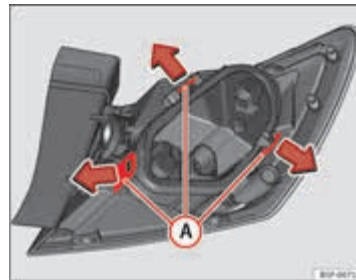
Afbeelding 153 Bevestigingslippen achter op achterlicht
