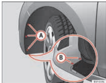
Afbeelding 148 Mistlamp: toegang tot de stekker en de lamphouder
