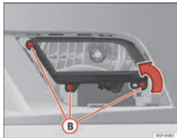
Afbeelding 147 Mis- tlamp
