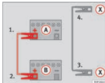
Afbeelding 132 Verbindingschema voor wagens met Start-stop-systeem.
