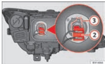
Afbeelding 140 Dimlicht
