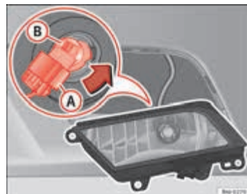
Afbeelding 150 Mistlamp
