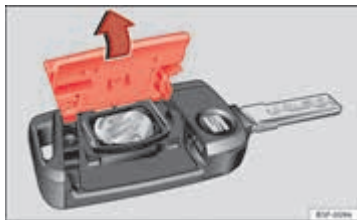
Afbeelding 48 Autosleutel: openen van het deksel van batterijcompartiment.
