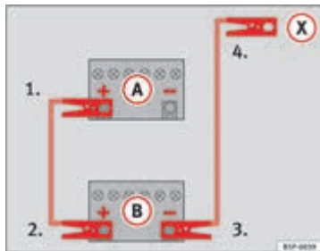
Afbeelding 131 Verbindingschema voor wagens zonder Start-stop-systeem.
