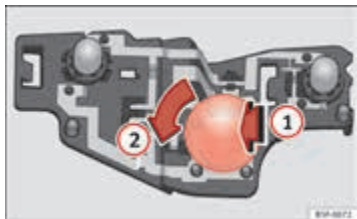
Afbeelding 156 Positie van de lampjes op de fitting.
