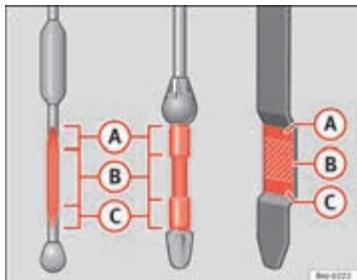
Afbeelding 113 Oliepeilstok
