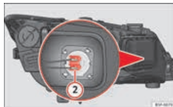
Afbeelding 145 Lampje van het grootlicht
