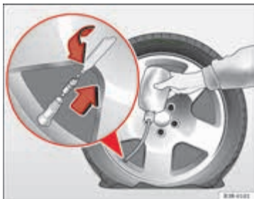
Afbeelding 123 Bandvullen
