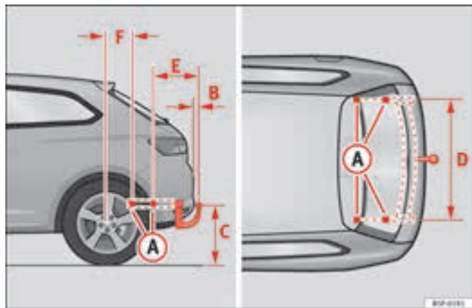
Afbeelding 110 Bevestigingspunten voor de trekhaak
