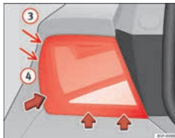
Abbeelding 152 Uitbouwen van achterlicht in zijpaneel
