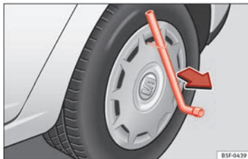
Afb. 69 Grote wioldop verwijderen.
