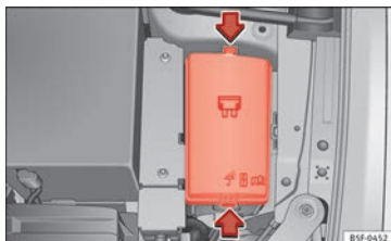
Afb. 101 In de motorruimte: deksel van de zekeringenhouder.
