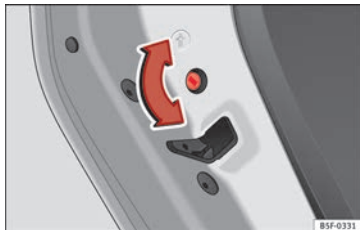
Afb. 134 Kinderslot in het linkerportier.
