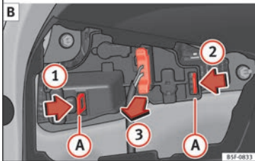
Afb. 113 Afdekking in de achterklep verwijderen en fitting demonteren.
