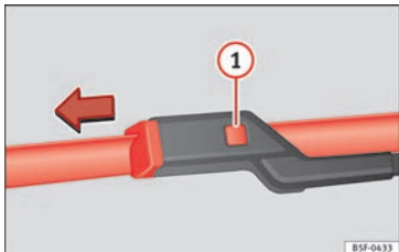
Afb. 80 Ruitenwischerbladen voorruit vervangen.
