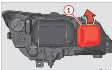
Afb. 105 Lampje knipperlicht.
