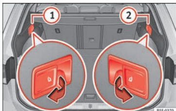
Afb. 152 In de bagageruimte: hendels voor de ontgrendeling op afstand van de linkerzijde ① en rechterzijde ② van de achterste rugleuning.
