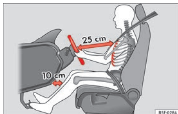
Afb. 82 De juiste afstand van de bestuurder tot het stuurwiel.
