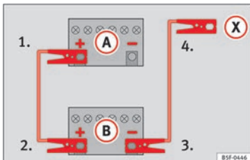
Afb. 77 Verbindingsschema voor wagens zonder Start-stopsysteem.
