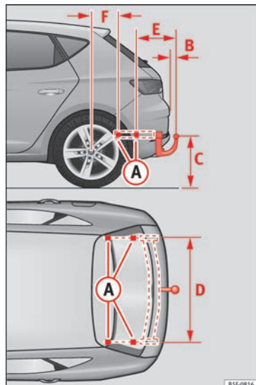
Afb. 238 Bepaling van de bevestigingspunten voor de trekhaak.
