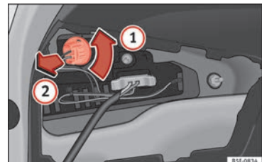
Afb. 116 Fitting uitbouwen. »
