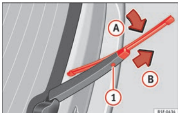
Afb. 81 Ruitenwischerblad van achterraut vervangen.
