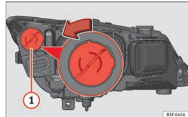
Afb. 104 Lampje van het daglicht.
