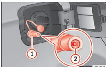
Afb. 239 Tankklep open: gasvulmond ①, plug van vulmond ②.
