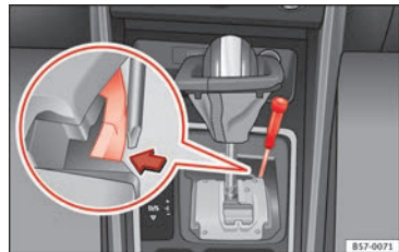
Afb. 54 Keuzehendel noodontgrendelen uit parkeerstand.
