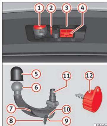
Afb. 225 Steun van de trekhaak voor aanhanger / afneembare kogelkop / sleutel
