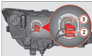
Afb. 103 Dimlicht.
