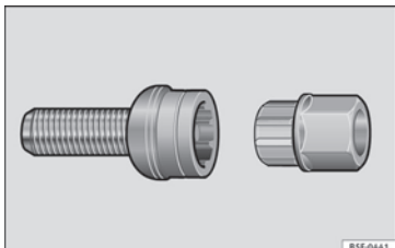
Afb. 71 Wielbout met diefstalbeveiliging, voorzien van dop en adapter.
