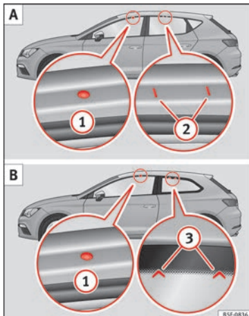
Afb. 183 Leon/Leon SC: bevestigingspunten voor de reling van het dakdragersysteem.
