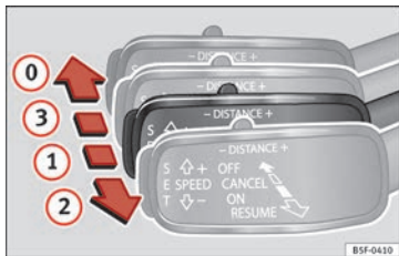
Afb. 200 Links van de stuurkolom: derde hendel om de automatische afstandsregeling te bedienen.
