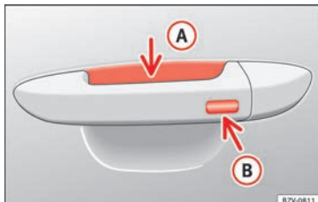
Afb. 131 Sluit- en startsysteem zonder sleutel Keyless Access: sensoroppervlak A voor het ontgrendelen aan de binnenzijde van de portiergreep van het portier en sensoroppervlak B voor het vergrendelen aan de buitenzijde van de portiergreep.
