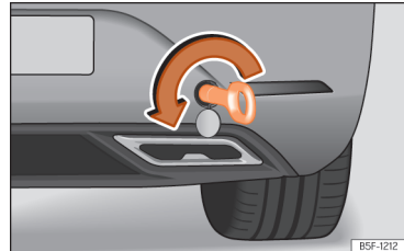
Afb. 214 Aan de rechterzijde van de achterbumper: vastgeschroefd sleepoog.
