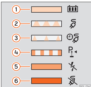
Afb. 61 Aan de binnenkant van de klep van de laadaansluiting: sticker met informatie over de indicator van het laadproces.
