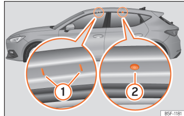
Afb. 195 Bevestigingspunten voor de reling van het dakdragersysteem (Leon).
