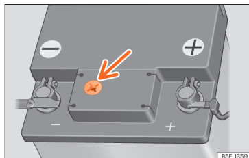
Afb. 230 Kijkglas aan de bovenzijde van de 12 volt-accu (schematische voorstelling).
