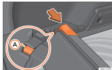
Afb. 180 In de bagageruimte: houder voor het bewaren van de oprolbare plank.
