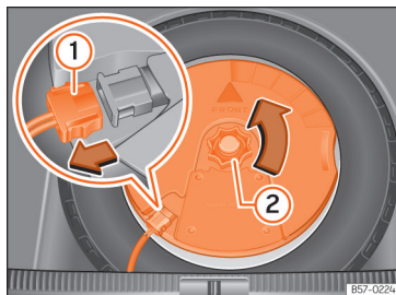
Afb. 236 In de bagageruimte: subwoofer uitbouwen.
