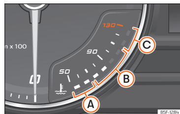
Afb. 10 Analoog instrumentenpaneel: koelvloeistoftemperatuurmeter.
