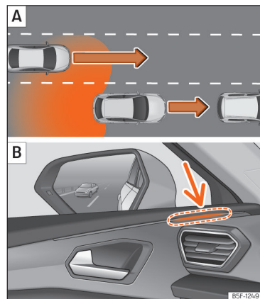
Afb. 144 Schematische weergave: A Inhalen met verkeer aan de achterzijde. B Indicatie van de rijstrookwisselassistent aan de linkerkzijde.
