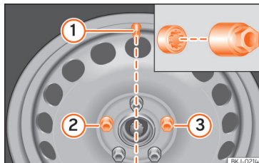
Afb. 241 Wiel verwisselen: ventiel van de band ① en montageplaats van de antidiefstalbout ② of ③.
