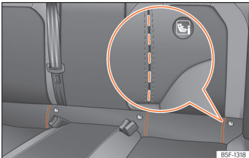
Afb. 44 Achterstoel: gestanste gleuven voor toegang tot de ISOFIX/i-Size-bevestigingsbeugels.
