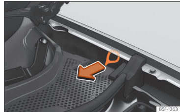
Afb. 62 Tussen het spatscherm links en het scharnier van de motorkap: Hendel voor handmatige noodontgrendeling van de laadsteker.
