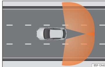
Afb. 126 Detectiegebieden van de sensoren.
