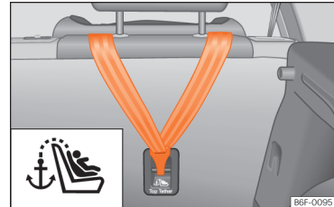
Afb. 49 Achterzijde van de achterstoelen: bevestigingsogen voor de Top Tether-riem.
