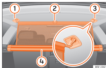
Afb. 183 In de bagageruimte: scheidingsnet inhaken.
