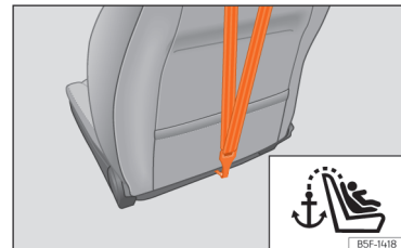
Afb. 50 Achterzijde van de rugleuning van de bijrijdersstoel: verankerung voor de Top Tether-riem.
