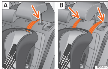
Afb. 47 Stoelen achterin: afstelling en montage volgens de Top Tether-gordel.
