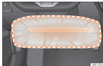
Afb. 40 Aan de bestuurderszijde: werkinggebied van de airbag voor de knieën.
