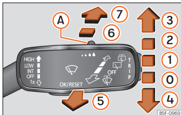
Afb. 105 Bediening van de ruitenwisser en ruitensproeier.
