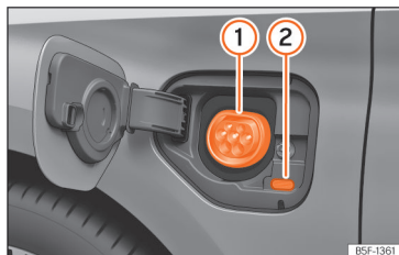
Afb. 59 Achter de laadklep van de accu linksvoor: Laadcontactdoos.
