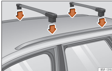
Afb. 194 Bevestigingspunten voor de reling van het dakdragersysteem [Leon Sportstourer].
