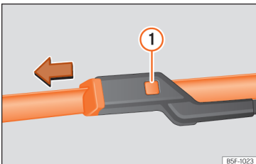
Afb. 208 Ruitenwisserbladen voorruit vervangen.
