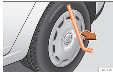
Afb. 237 Grote wioldop verwijderen.
