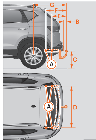
Afb. 214 Maten en bevestigingspunten voor het achteraf inbouwen van een trekhaak.
