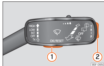
Afb. 76 Ruitenwisserhandel: bedieningstoetsen.
