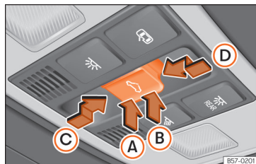
Afb. 104 In de hemelbekleding: knop van het glazen dak.
