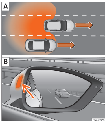
Afb. 191 Schematische weergave: A Situatie van het inhalen en daarna opnieuw invoegen in de rechter rijstrook. B Indicatie van de rijstrookwisselassistent in de buitenspiegel rechts.
