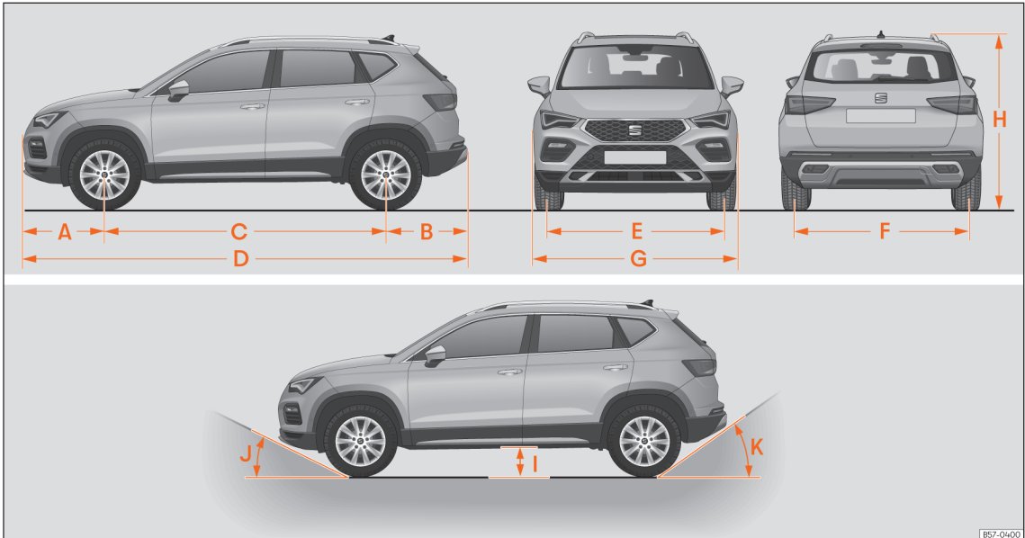
Afb. 233 Afmetingen
