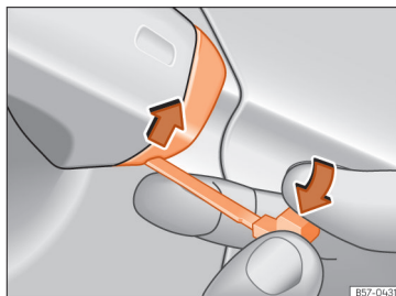
Afb. 94 Portiergreep aan bestuurderszijde: klep losmaken door los te wippen.
