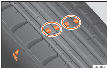
Afb. 228 Bandenprofiel: slijtagemerkttekens.
