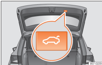
Afb. 98 Achterklep: toets om de klep te sluiten.
