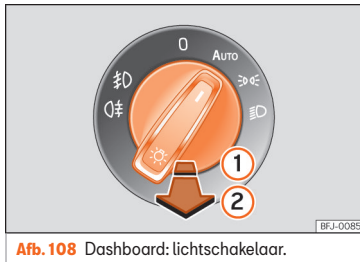
Afb. 108 Dashboard: lichtschakelaar.
