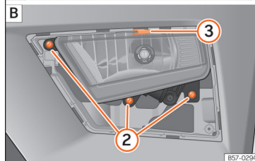
Afb. 57 Mistlamp: rooster verwijderen.
