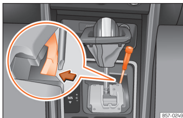
Afb. 164 Keuzehendel: noodontgrendeling in de parkeerstand.
