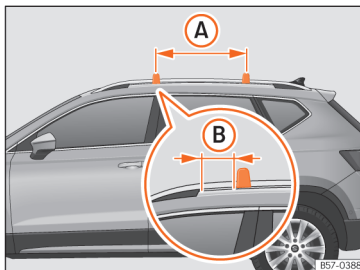
Afb. 139 Bevestigingspunten voor de reling van het dakdragersysteem.
