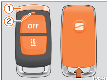
Afb. 148 Interieurvoorverwarming: radiografische afstandsbediening.
