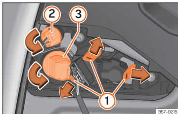
Afb. 62 Fitting uitbouwen.
