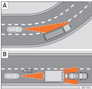
Afb. 182 A Wagen in een bocht. B Motorrijder die voor u rijdt, buiten de actieradius van de radarsensor.
