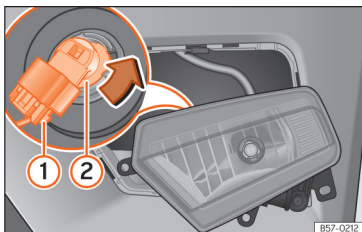
Afb. 58 Mistlamp: fitting uitbouwen
