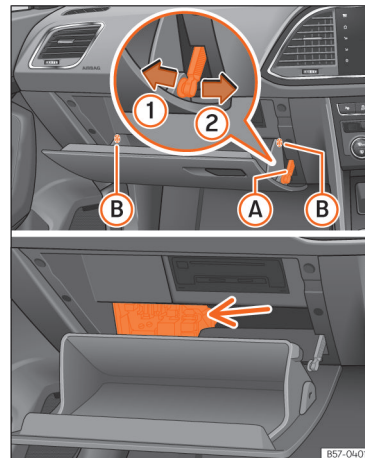
Afb. 50 Dashboardkastje (stuur rechts): toegang tot de zekeringenhouder.
