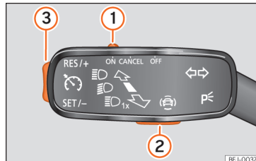
Afb. 175 In de knipperlichthendel: toetsen voor bediening van de snelheidsbegrenzer.
