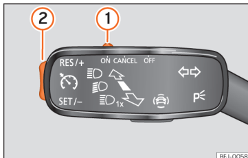
Afb. 173 In de knipperlichthendel: bedieningselementen voor SRS.
