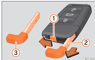
Afb. 86 Wagensleutel: de nood sleutel verwijderen.
