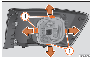
Afb. 60 Bevestigingslippen aan de achterzijde van het achterlicht.
