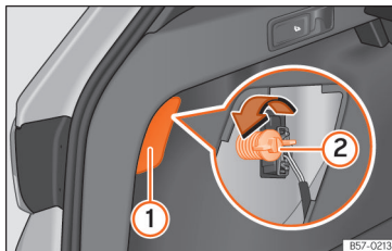
Afb. 59 Bagageruimte: toegang tot de bevestigingsbout van het achterlicht.
