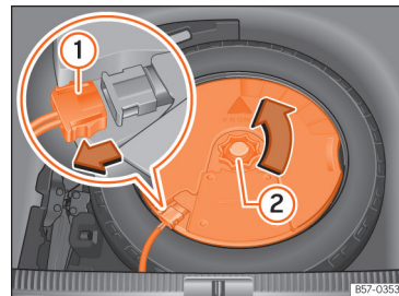
Afb. 223 In de bagageruimte: subwoofer uitbouwen.
