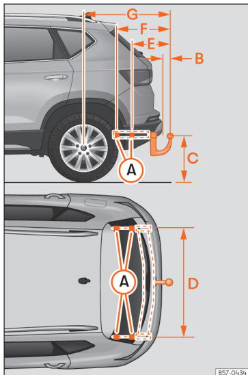
Afb. 203 Maten en bevestigingspunten voor het achteraf inbouwen van een trekhaak.
