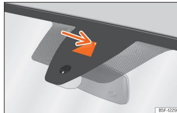
Afb. 159 Op de voorruit: gezichtsveld van de rijstrookassistent.
