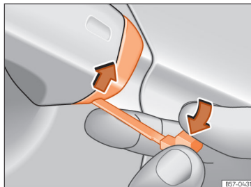
Afb. 83 Portiergreep aan bestuurderszijde: klep losmaken door los te wippen.
