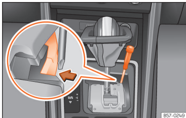
Afb. 155 Keuzehendel: noodontgrendeling in de parkeerstand.
