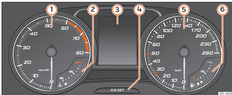
Afb. 54 Instrumentenpaneel, in het dashboard.
