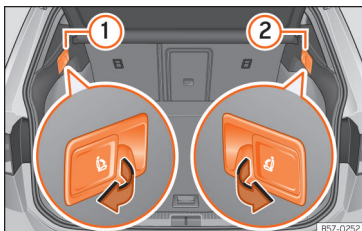
Afb. 113 In de bagageruimte: hendels voor de ontgrendeling op afstand van de linkerzijde ① en rechterzijde ② van de achterste rugleuning.
