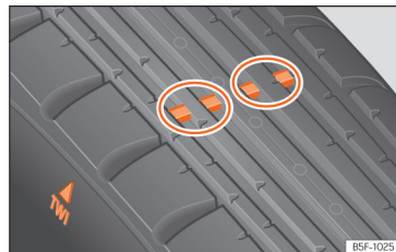
Afb. 219 Bandenprofiel: slijtagemerkttekens.
