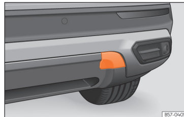
Afb. 195 Aan de rechterzijde van de achterbumper: de afdekking verwijderen.
