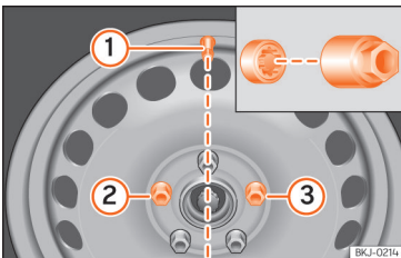
Afb. 223 Wiel verwisselen: ventiel van de band ① en montageplaats van de antidiefstalbout ② of ③.
