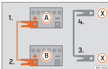
Afb. 192 Verbindingschema voor wagens met Start-stopsysteem.
