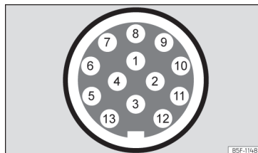
Afb. 179 Schematische weergave: toewijzing van de pinnen van het stopcontact voor de aanhangwagen.
