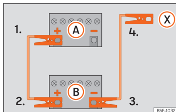
Afb. 191 Verbindingschema voor wagens zonder Start-stopsysteem.
