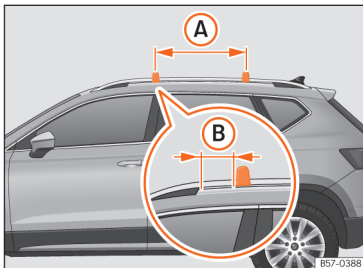
Afb. 178 Bevestigingspunten voor de reling van het dakdragersysteem
