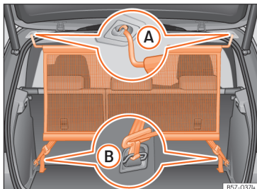
Afb. 171 Scheidingsnet gemonteerd.
