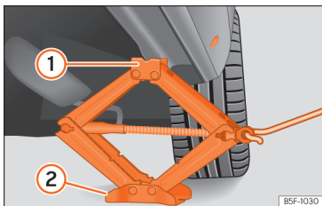
Afb. 225 Langsligger: plaatsing van de wagenkrik.
