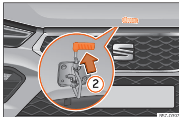
Afb. 201 Hendel onder de motorkap.
