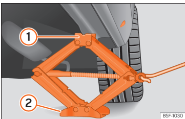
Afb. 222 Langsligger: plaatsing van de wagenkrik.
