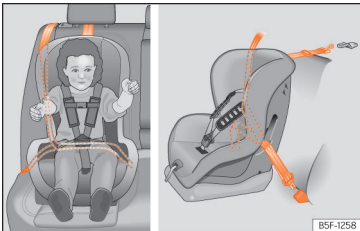
Afb. 43 Op de achterbank: inbouw van het kindersitje.
