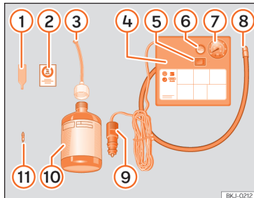
Afb. 224 Standaardweergave: inhoud van de bandenafdichtset.
