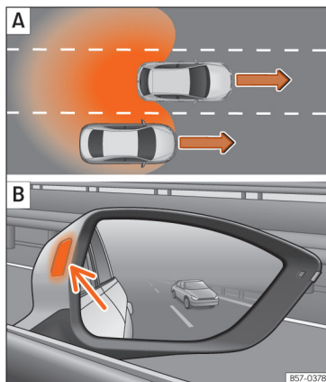
Afb. 129 Schematische weergave: A Inhalen op de middelste rijstrook en daarna opnieuw invoegen in de rechter rijstrook. B Indicatie van de rijstrookwisselassistent aan de rechterzijde.
