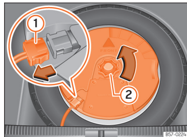
Afb. 215 In de bagageruimte: subwoofer uitbouwen.
