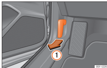
Afb. 200 Ontgrendelingshendel in de voetenruimte van de bestuurder.
