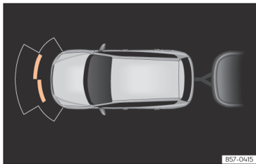
Afb. 133 Weergave van de parkeerhulp op het scherm met aangekoppelde aanhangwagen.
