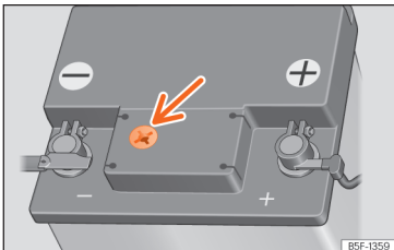
Afb. 210 Kijkglas aan de bovenzijde van de 12 volt-accu (schematische voorstelling).
