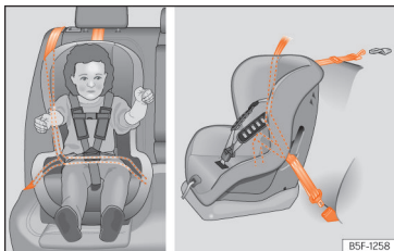
Afb. 29 Op de achterstoelen: inbouw van het kindersitje.
