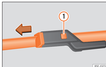
Afb. 41 Ruitenwischerbladen voorruit vervangen.
