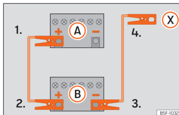
Afb. 42 Verbindingsschema voor wagens zonder start-stopsysteem.
