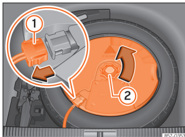
Afb. 194 In de bagageruimte: subwoofer uitbouwen.
