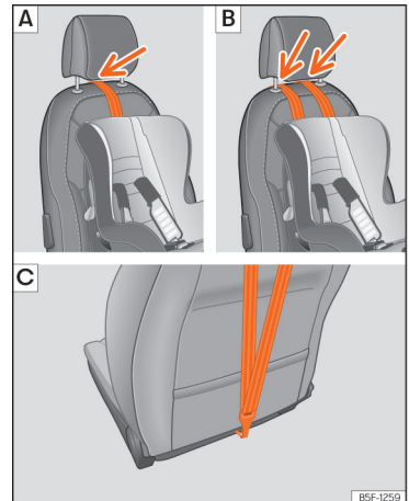
Afb. 28 Bijrijdersstoel: afstelling en montage volgens de Top Tether-gordel.
