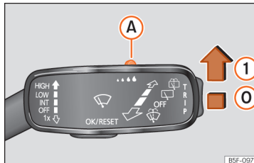
Afb. 90 Ruitenswisserhendel: regensensor A afstellen.
