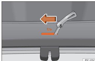
Afb. 80 Detail van de bagageruimte: noodontgrendeling.
