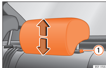
Afb. 96 Hoofdsteun achterin: regeling van de hoofdsteun.
