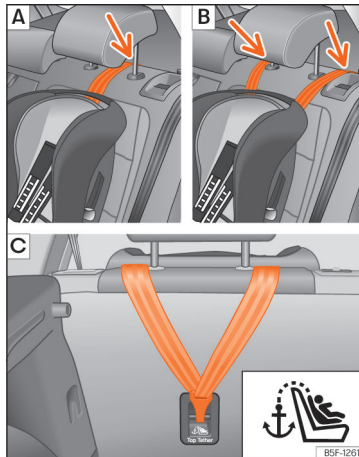
Afb. 27 Zitplaatsen achterin: afstelling en montage volgens de Top Tether-gordel.
