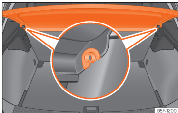
Afb. 102 In de bagageruimte: hoedenplank uit- en inbouwen.
