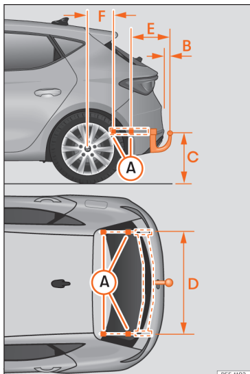
Afb. 176 Maten en bevestigingspunten voor het achteraf inbouwen van een trekhaak.
