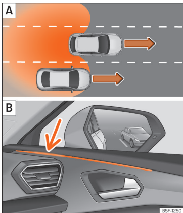
Afb. 159 Schematische weergave: A Situatie van het inhalen op de middelste rijstrook en daarna opnieuw invoegen in de rechter rijstrook. B Indicatie van de rijstrookwissel in het controlelampje aan de rechterzijde.
