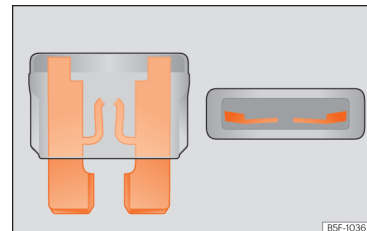
Afb. 50 Voorbeeld van een doorgebrande zekering.
