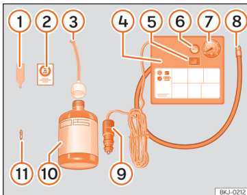
Afb. 39 Standaardweergave: inhoud van de bandenafdichtset.
