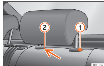
Afb. 115 Hoofdsteun achterin: verwijderen.
