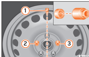
Afb. 44 Wiel verwisselen: ventiel van de band ① en montageplaats van de antidiefstalbout ② of ③.
