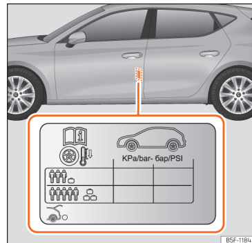
Afb. 234 Plaats van de sticker van de bandenspanningen.
