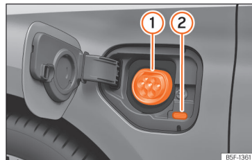
Afb. 210 Achter de laadklep van de accu linksvoor: Laadstopcontact
