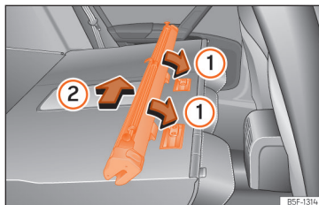
Afb. 140 Scheidingsnet op de rugleuningen van de achterbank inbouwen.
