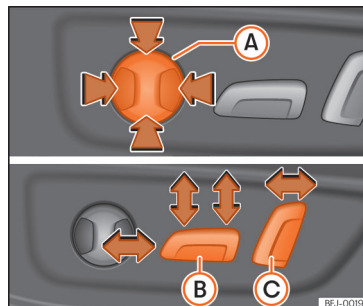
Afb. 112 Bestuurdersstoel: elektrische instelling van de stoel.
