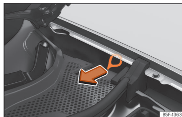
Afb. 213 Tussen het spatscherm links en het scharnier van de motorkap: Hendel voor handmatige noodontgrendeling van de laadstekker.
