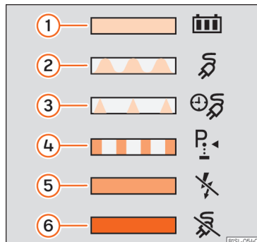
Afb. 212 Aan de binnenkant van de acculaadklep: sticker met informatie over de laadprocesindicatie.
