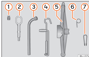
Afb. 38 Onder de afdekking van de laadvloer van de bagageruimte:: wagengereedschap.
