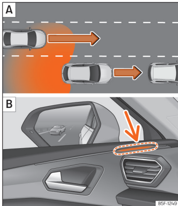
Afb. 190 Schematische weergave: A ) Situatie van het inhalen met verkeer aan de achterzijde. B ) Indicatie van de rijstroomwisselhelp in het controlelampje aan de linkerzijde.
