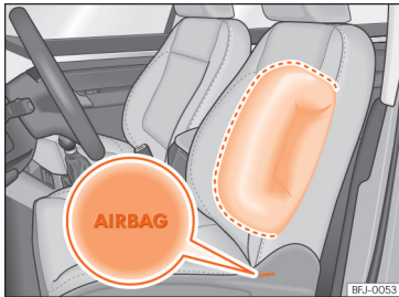
Afb. 26 Zij-airbag in de bestuurdersstoel.
