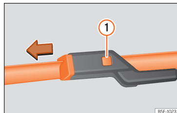
Afb. 48 Ruitenwischerbladen voorruit vervangen.
