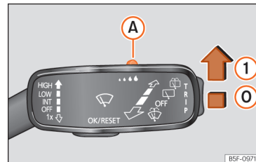
Afb. 108 Ruitenwisherhendel: regensensor afstellen.
