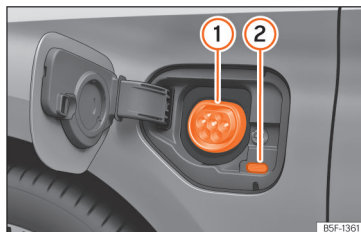
Afb. 213 Achter de laadklep van de accu linksvoor: Laadcontactdoos
