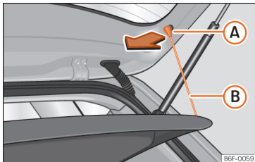
Afb. 122 In de bagageruimte: hoedenplank uit- en inbouwen.
