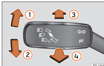
Afb. 103 Knipperlicht- en grootlichthendel.
