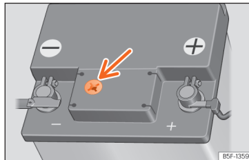
Afb. 238 Kijkglas aan de bovenzijde van de 12 volt accu (schematische voorstelling).
