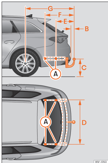
Afb. 208 Maten en bevestigingspunten voor het achteraf inbouwen van een trekhaak.
