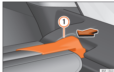
Afb. 127 In de bagageruimte: hoedenplank uitbouwen.
