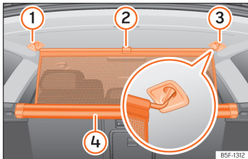
Afb. 139 In de bagageruimte: scheidingsnet inhaken.
