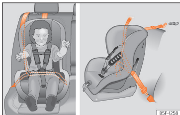
Afb. 51 Op de achterbank: inbouw van het kinderzitje.
