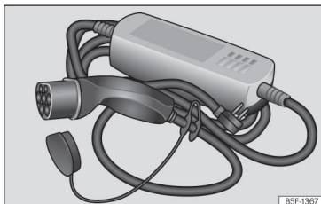
Afb. 64 Laadkabel voor stopcontacten.
