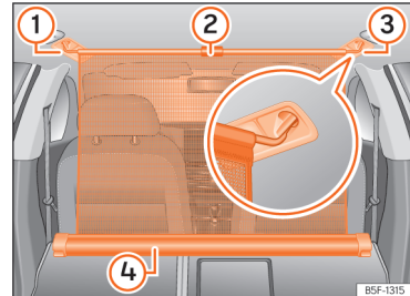
Afb. 187 In de bagageruimte: scheidingsnet vastgehaakt met neergeklapte rugleuningen van de achterbank.
