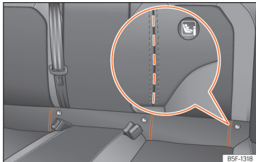
Afb. 44 Achterstoel: gestante gleuven voor toegang tot de ISOFIX/i-Size-bevestigingsbeugels.
