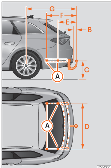
Afb. 201 Maten en bevestigingspunten voor het achteraf inbouwen van een trekhaak.
