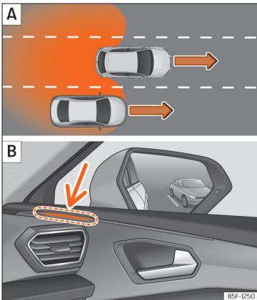
Afb. 146 Schematische weergave: A Inhalen op de middelste rijstrook en daarna opnieuw invoegen in de rechter rijstrook. B Indicatie van de rijstrookwisselassistent aan de rechterzijde.
