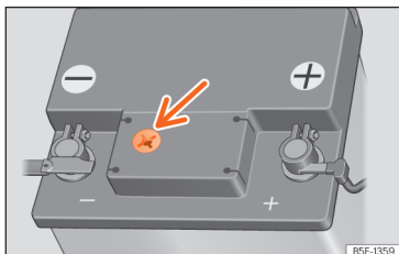
Afb. 231 Kijkglas aan de bovenzijde van de 12 volt-accu (schematische voorstelling).
