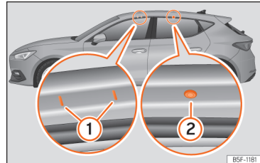
Afb. 196 Bevestigingspunten voor de reling van het dakdragersysteem (Leon).
