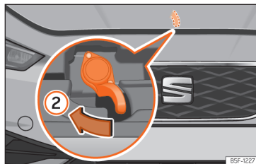
Afb. 220 Hendel onder de motorkap.
