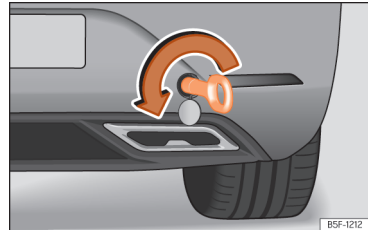
Afb. 215 Aan de rechterzijde van de achterbumper: vastgeschroefd sleepoog.
