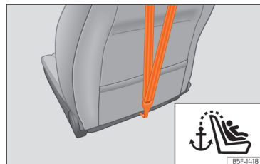
Afb. 50 Achterzijde van de rugleuning van de bijrijdersstoel: verankerung voor de Top Tether-riem.
