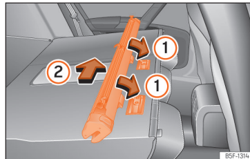
Afb. 186 Scheidingsnet op de rugleuningen van de achterbank inbouwen.
