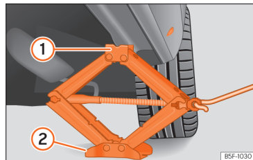
Afb. 244 Langsligger: plaatsing van de wagenkrik.
