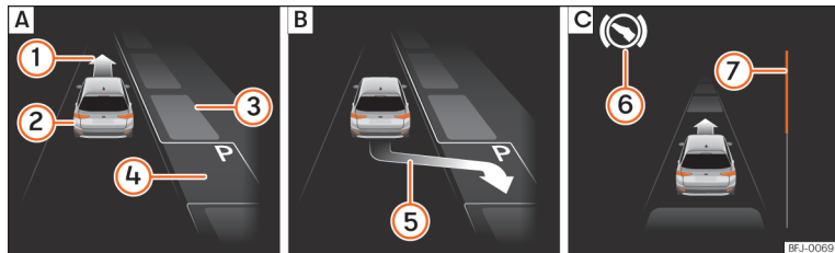
Afb. 284 Op het display van het instrumentenpaneel: recht parkeren. [A] Een parkeerplaats zoeken. [B] Positie om te parkeren. [C] Manoeuvreren.
