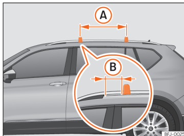
Afb. 138 Bevestigingspunten voor de reling van het dakdragersysteem.
