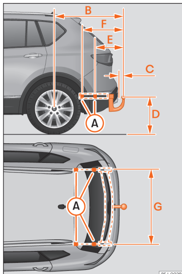
Afb. 304 Maten en bevestigingspunten voor het achteraf inbouwen van een trekhaak.
