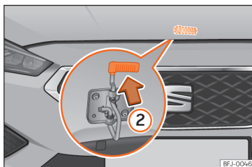
Afb. 311 Hendel onder de motorkap.
