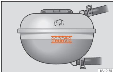
Afb. 315 In de motorruimte: markering aan het koelvloeistofexpansiereservoir.
