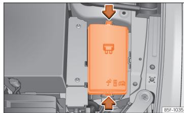
Afb. 54 In de motorruimte: afdekking van de zekeringenhouder.
