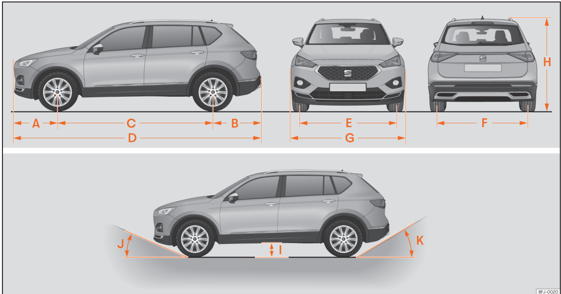
Afb. 325 Afmetingen
