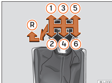
Afb. 244 Schakelschema van handgeschakelde 6-versnellingsbak.
