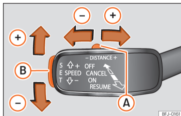
Afb. 266 Links van de stuurkolom: derde hendel voor bediening van ACC.
