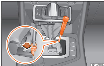
Afb. 248 Keuzehendel: noodontgrendeling in de parkeerstand.
