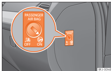
Afb. 18 Sleutelschakelaar voor het in- en uitschakelen van de bijrijdersairbag.
