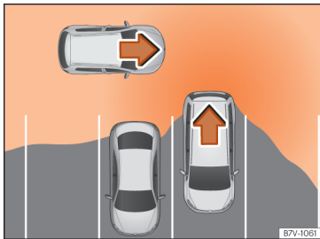
Afb. 277 Schematische weergave van de uitparkeerhulp: bewaakte zone rond de wagen die aan het uitparkeren is.
