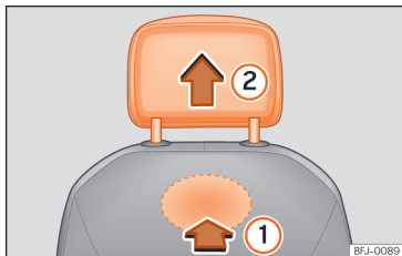
Afb. 113 Voorste hoofdsteun: verwijderen.
