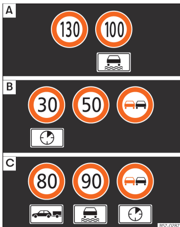
Afb. 61 Op het display van het instrumentenpaneel: voorbeelden van herkende snelheidsbeperkingen of inhaalverboden met de overeenkomstige aanvullende borden.
