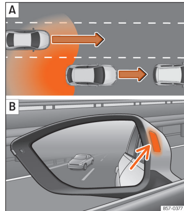
Afb. 196 Schematische weergave: A Situatie van het inhalen met verkeer aan de achterzijde. B Indicatie van de rijstrookwisselassistent in de buitenspiegel links.
