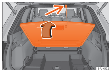
Afb. 123 In de bagageruimte: verstelbare bodem optillen.
