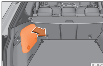
Afb. 248 Inbouwplaats van de accu in de bagageruimte
