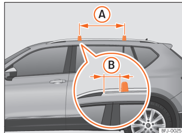
Afb. 133 Bevestigingspunten voor de reling van het dakdragersysteem.
