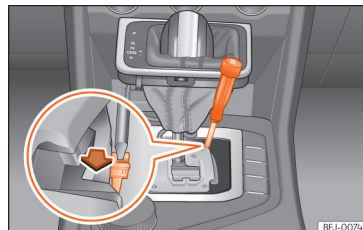
Afb. 169 Keuzehendel: noodontgrendeling in de parkeerstand.
