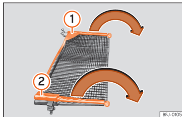
Afb. 130 Scheidingsnet uitklappen.
