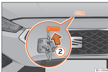
Afb. 239 Hendel onder de motorkap.
