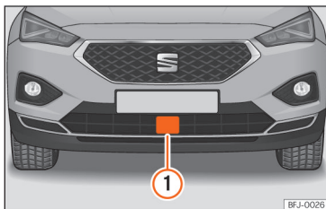
Afb. 172 In de voorbumper: radarsensor.
