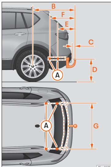
Afb. 221 Maten en bevestigingspunten voor het achteraf inbouwen van een trekhaak.
