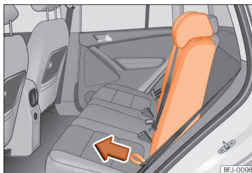
Afb. 114 Rugleuning achterstoel neer- en terugklappen.
