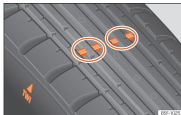
Afb. 251 Bandenprofiel: slijtagemerktkens.
