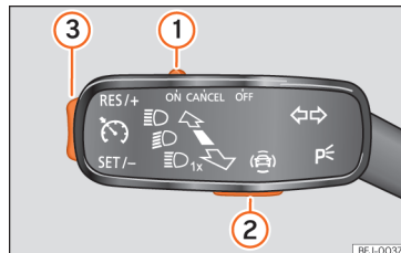
Afb. 181 In de knipperlichthendel: toetsen voor bediening van de snelheidsbegrenzer.
