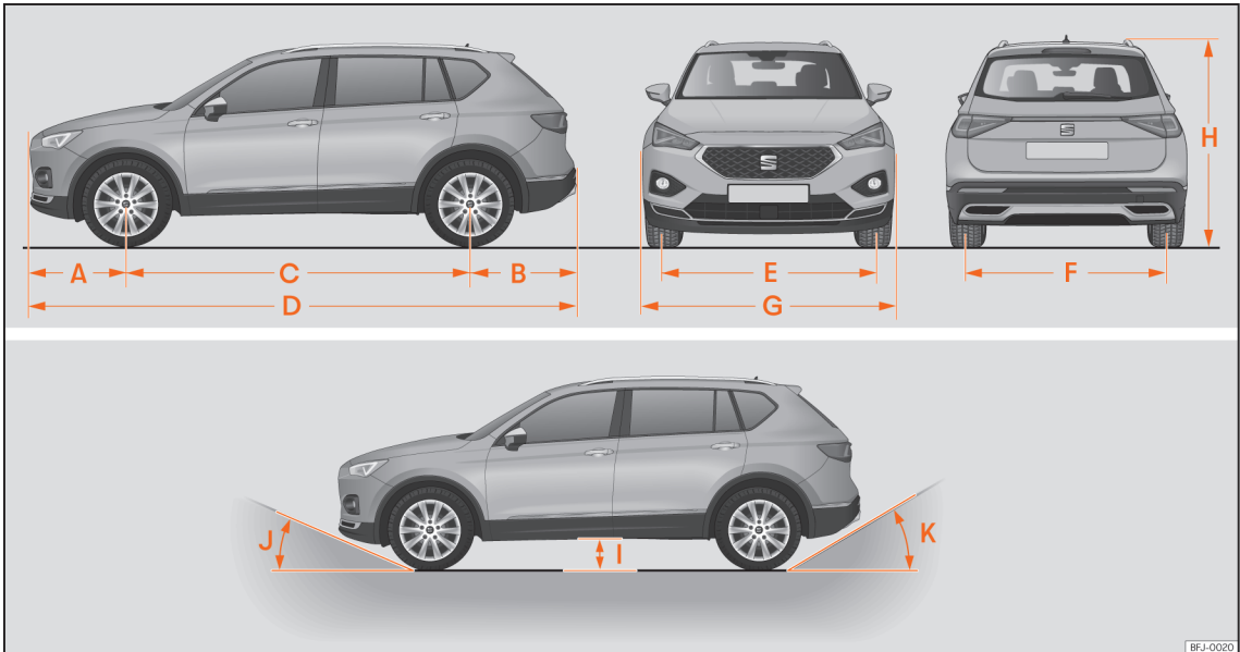
Afb. 256 Afmetingen
