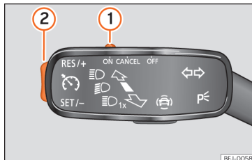
Afb. 179 In de knipperlichthendel: bedieningselementen voor SRS.
