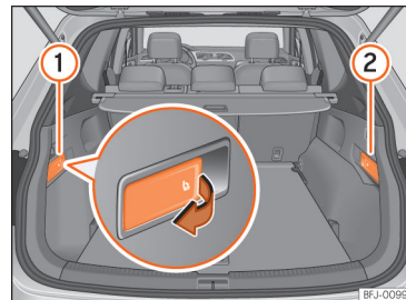
Afb. 115 In de bagageruimte: hendels voor de ontgrendeling vanaf de bagageruimte van de linkerzijde ① en rechterzijde ② van de achterste rugleuning.
