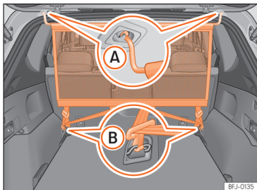
Afb. 132 Scheidingsnet gemonteerd.
