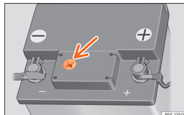
Afb. 249 Kijkglas aan de bovenzijde van de 12 volt accu (schematische voorstelling).
