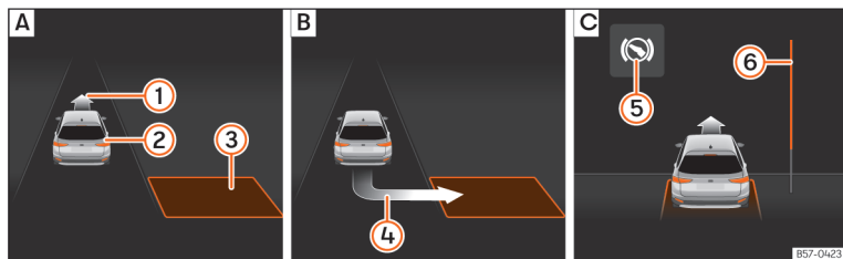
Afb. 205 Op het display van het instrumentenpaneel: schuin parkeren. [A] Een parkeerplaats zoeken. [B] Positie om te parkeren. [C] Manoeuvreren.
