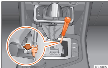
Afb. 170 Keuzehendel: noodontgrendeling in de parkeerstand.
