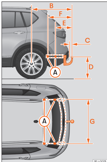
Afb. 220 Maten en bevestigingspunten voor het achteraf inbouwen van een trekhaak.
