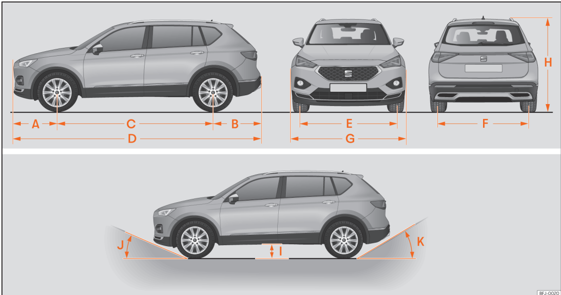
Afb. 257 Afmetingen
