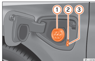
Afb. 226 Achter de laadklep van de accu linksvoor: Laadcontactdoos
