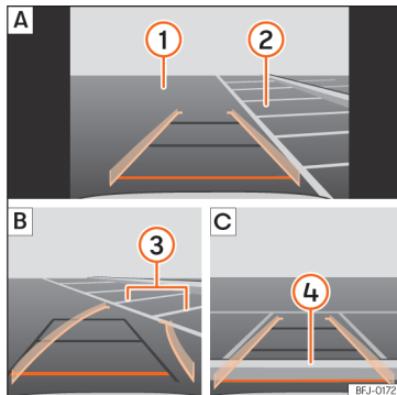
Afb. 216 Weergave op het beeldscherm van het infotainmentsysteem: parkeren met de achteruitrijhulp.
