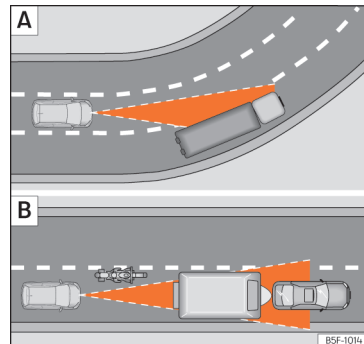
Afb. 187 [A] Wagen in een bocht. [B] Motorrijder die voor u rijdt, buiten de actieradius van de radarsensor. »
